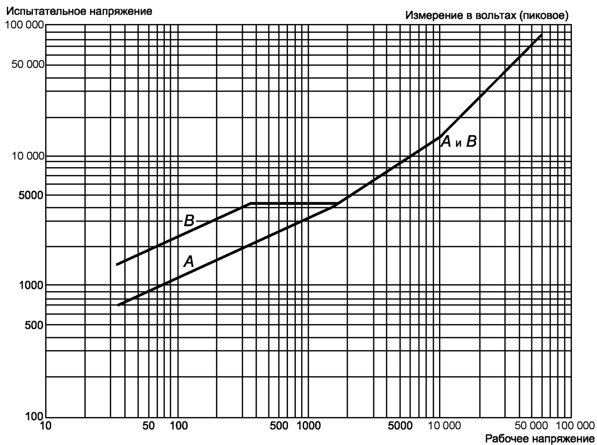
Рисунок PS-D.7 — Испытательные напряжения
