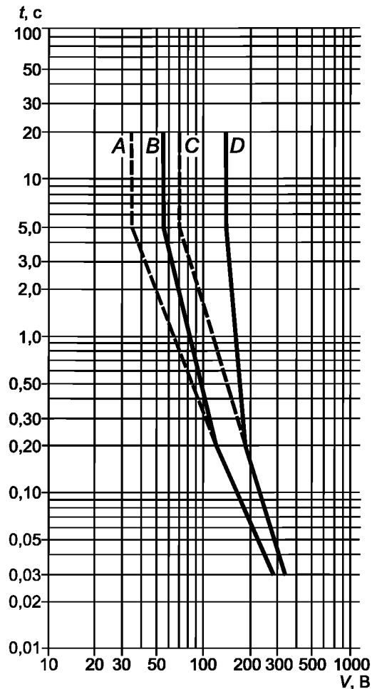
Рисунок PS-A.1 — Максимальная длительность кратковременных переходных доступных напряжений в условии первичного отказа [см. PS-A.6.3.2, перечисление а)]
