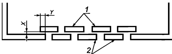
Рисунок PS-A.6 — Отражатель
