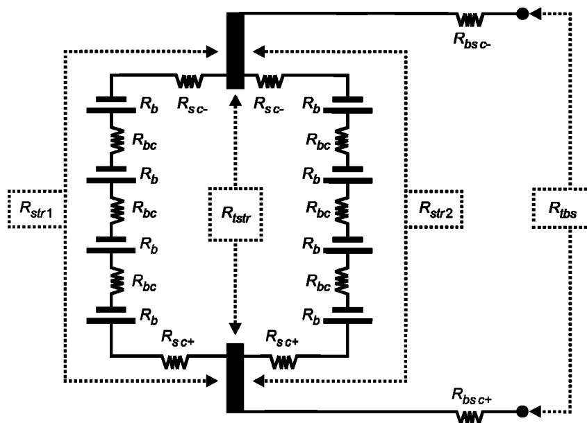
Рисунок PS-E.1.100.A — Расчеты сопротивления и короткого замыкания
