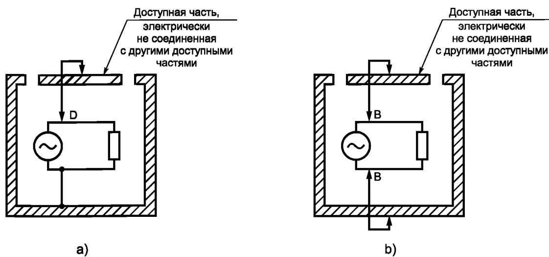
Рисунок D.2 a), b) — Защита между внутренней опасной для жизни цепью и доступной частью, не соединенной с другими доступными частями
