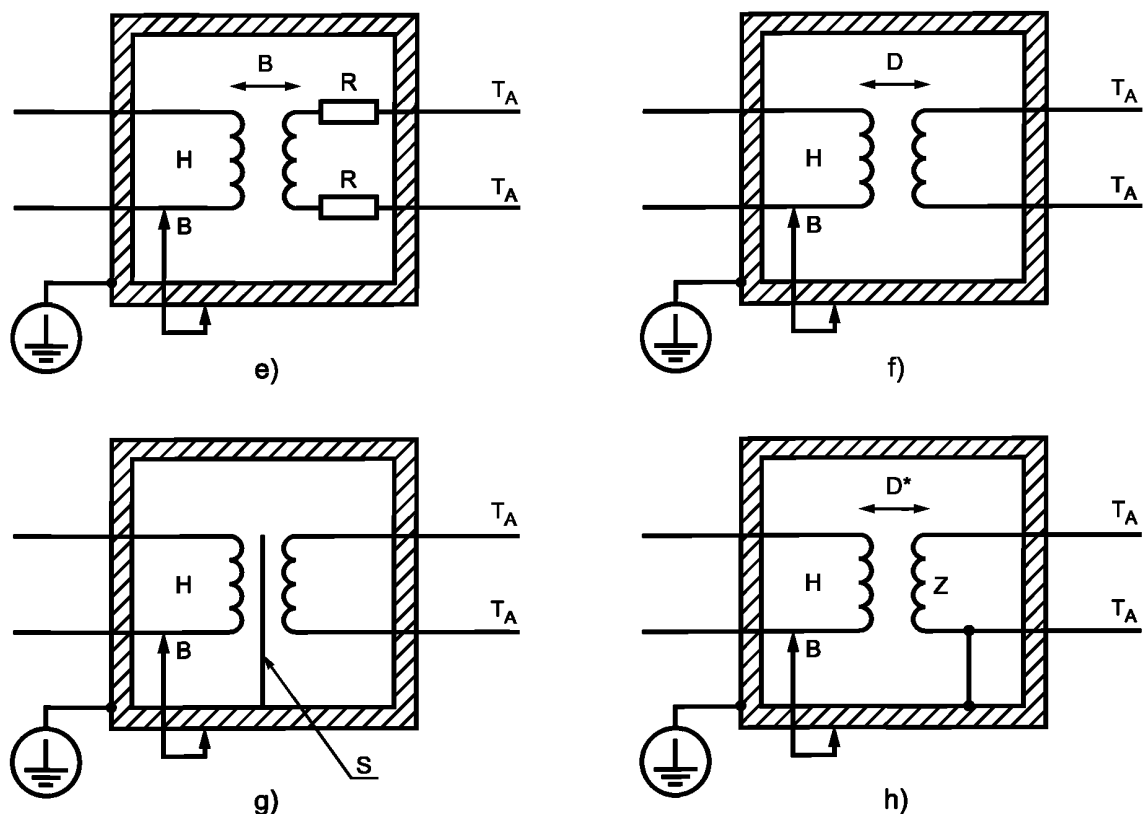
Рисунок D.1 e) — h) — Защита между опасными для жизни цепями и цепями, имеющими внешние клеммы на доступных частях
