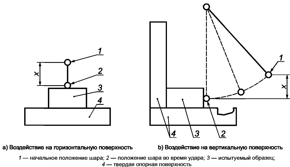
Рисунок 10 — Испытание на удар с помощью шара
