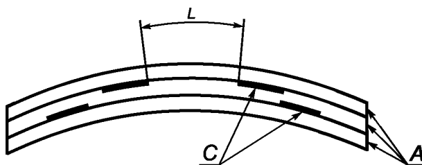
L — расстояние между соседними проводниками; A — слой тонкопленочного материала, например ленты полиэстерной пленки; C — проводники
