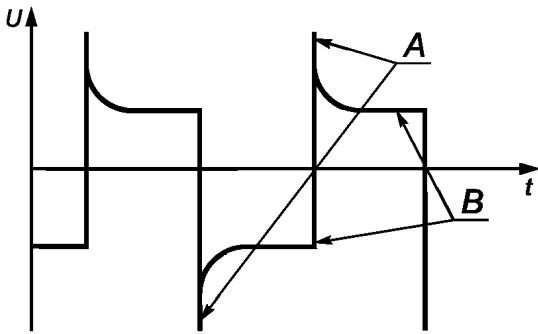
A — пиковое значение повторяющегося напряжения; B — значение рабочего напряжения
