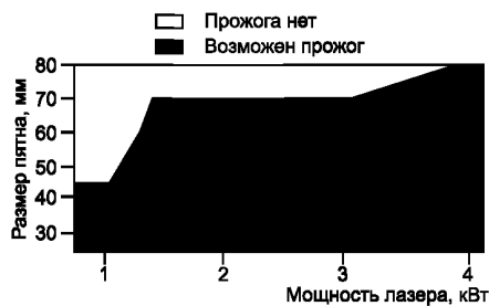
Рисунок F.14 — Стойкость к разрушению листа оцинкованной стали толщиной 1 мм от 100 с экспозиции расфокусированного пучка во время экспериментов с использованием непрерывного лазера на иттрий-алюминиевом гранате с неодимом
