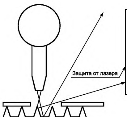
Рисунок В.3с — Отсутствие заготовки
