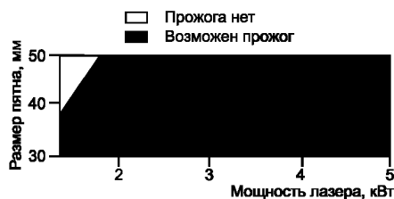
Рисунок F.12 — Стойкость к разрушению листа поликарбоната толщиной 6 мм от 100 с экспозиции расфокусированного пучка во время экспериментов с использованием непрерывного лазера на углекислом газе
