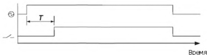
Рисунок 1 – Реле с задержкой по включению электропитания
