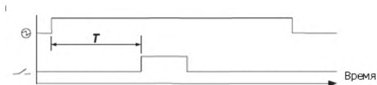
⊕ – источник электропитания; T – установленное время; ⚡ – главный контакт Рисунок 8 – Импульсное реле с задержкой
