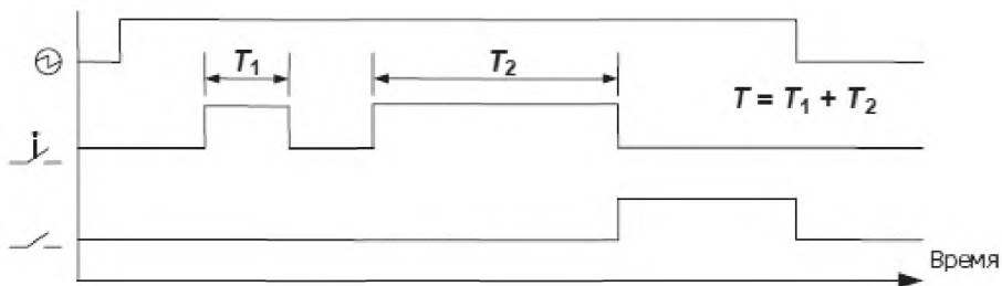
Рисунок 7 – Реле время суммирования
