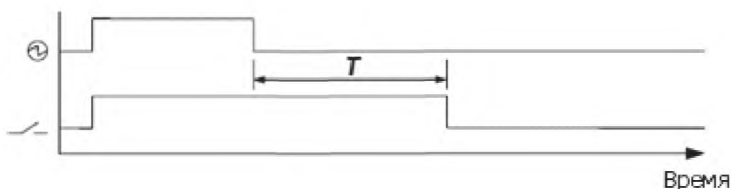
⊕ – источник электропитания; T – установленное время; — — — — — главный контакт Рисунок 2 – Реле с задержкой по выключению электропитания
