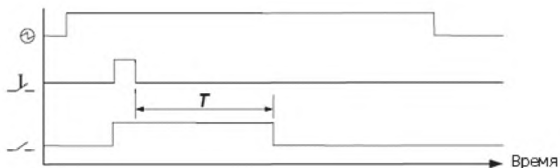
⊕ – источник электропитания; J – сигнал управления; T – установленное время; — — — — — главный контакт
