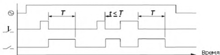
⊕ – источник электропитания; J – сигнал управления; T – установленное время; — – рабочий контакт
