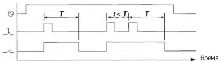
⊕ – источник электропитания; J – сигнал управления; T – установленное время; — – рабочий контакт
