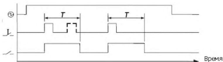
⊕ – источник электропитания; ⏏ – сигнал управления; T – установленное время; ⏏ – рабочий контакт
