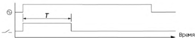
⊕ – источник электропитания; T – установленное время; ⏏ – рабочий контакт Рисунок 10 – Интервальное реле
