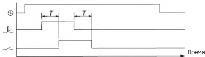
⊕ – источник электропитания; J – сигнал управления; T – установленное время; — — — — — главный контакт
