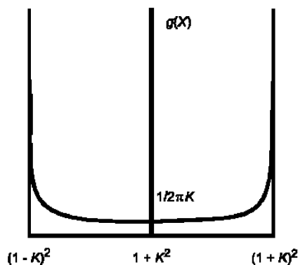
Рисунок 9 – U-образная ФПВ
