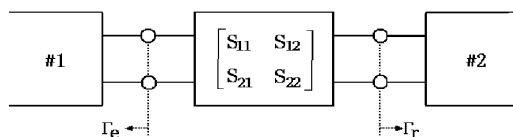
Рисунок 10 – Пример схемы
