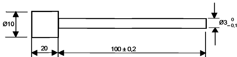
Рисунок 101 — Испытательный прут для скрытой блокировки
