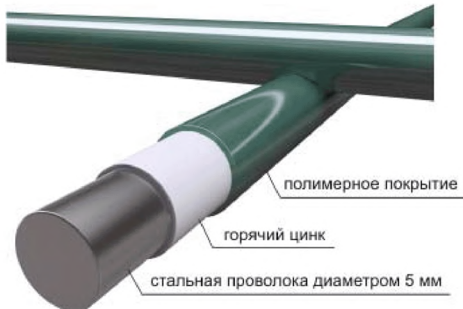
Рис. 1.2 - Противокоррозионное покрытие полотна.
