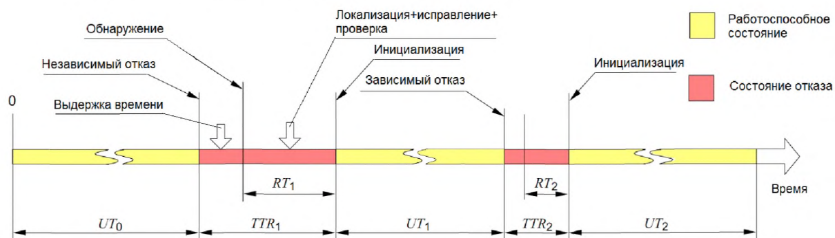
Рисунок С.2 — Схема обнаружения отказа
