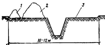
Рис. 43. Схема расположения грунта и рабочих мест при прокладке коммуникаций
