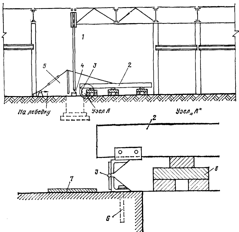
Рис. 25. Замена металлических колонн с помощью опорного шарнира
