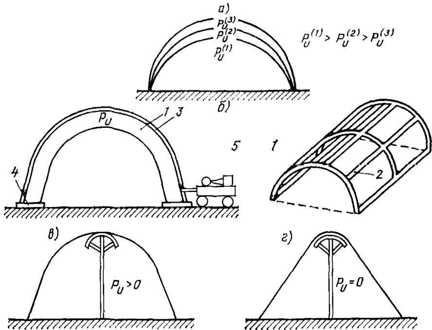
Рис. 9. Конструктивные схемы пневмосооружений
