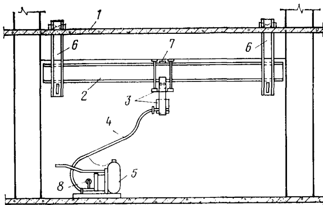
Рис. 42. Усиление железобетонной балки с помощью металлической
