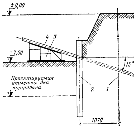
Рис. 13. Крепление стены котлована с помощью грунтовых анкеров
