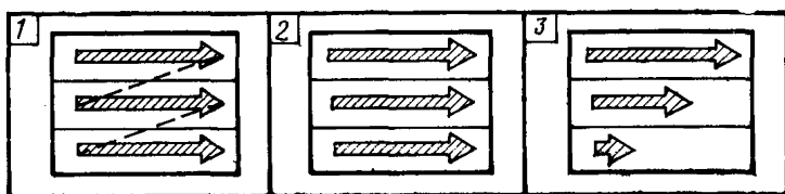
Рис. 31. Очередность выполнения монтажных работ при реконструкции многопролетных зданий
