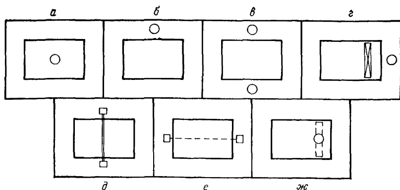
Рис. 28. Возможные варианты установки кранов при реконструкции пролетов
