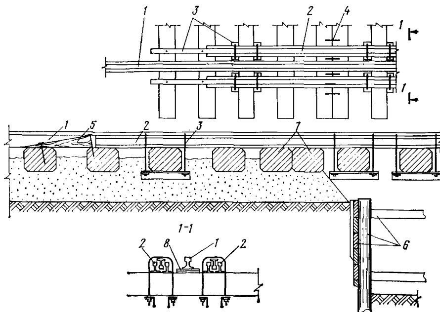
Рис. 46. Усиление железнодорожного пути над траншеей с помощью рельсовых пакетов
