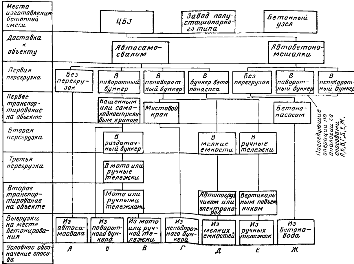
Рис. 19. Варианты процессов транспортирования и подачи бетонной смеси к месту бетонирования в условиях реконструкции
