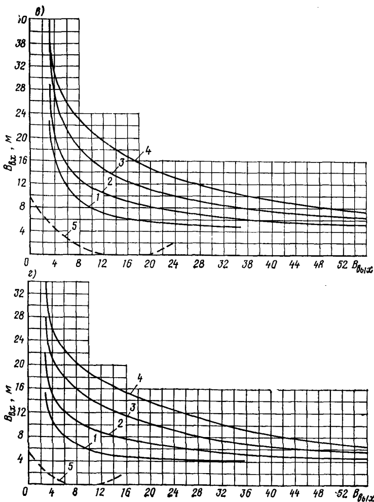
Рис. 27. Вписываемость в прямоугольный проезд седельных тягачей с полуприцепами
