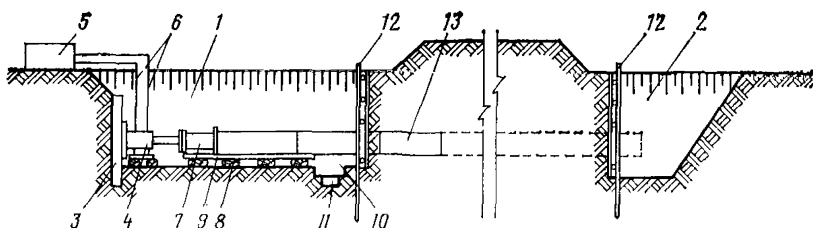
Рис. 47. Схема технологического процесса прокладки коммуникаций методом продавливания (прокальвания)
