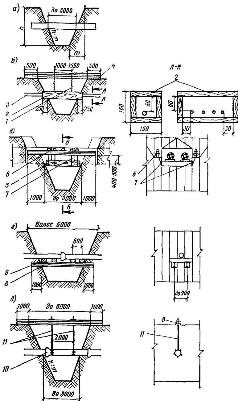
Рис. 44. Защита вскрываемых коммуникаций от механических повреждений
