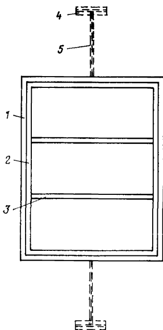
Рис. 12. Крепление котлована с помощью распорных рам и грунтовых анкеров
