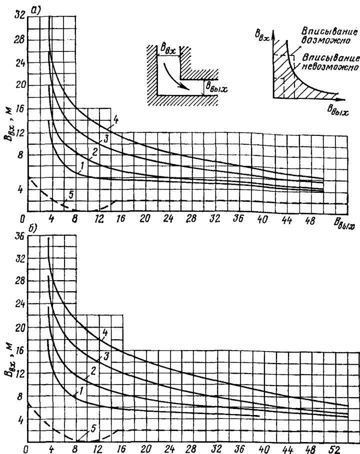
Рис. 26. Вписываемость в прямоугольный проезд седельных тягачей с полуприцепами
