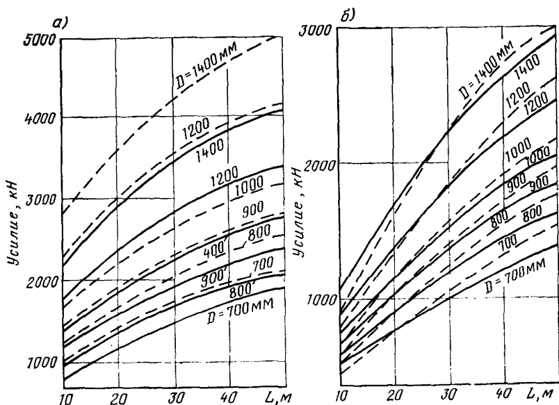
Рис. 48. График для определения усилий, требующихся для продавливания стальных футляров (пунктирная линия — для песчаных грунтов, сплошная — для глинистых)
