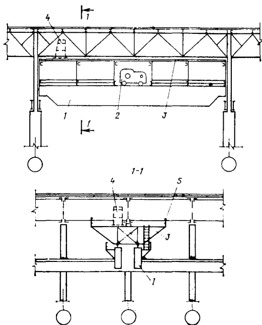
Рис. 34. Схема об- стройки мостово- го крана при уси- лении кровли
