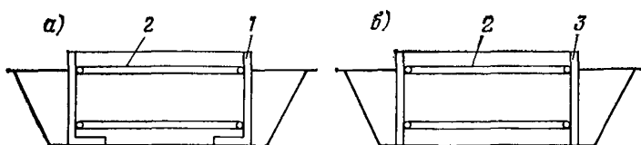
Рис. 18. Опалубка фундамента под оборудование из железобетона а — из элементов Г-образного сечения; б — из плоских плит; 1 — Г-образные элементы; 2 — распорные рамы; 3 — плоские плиты
