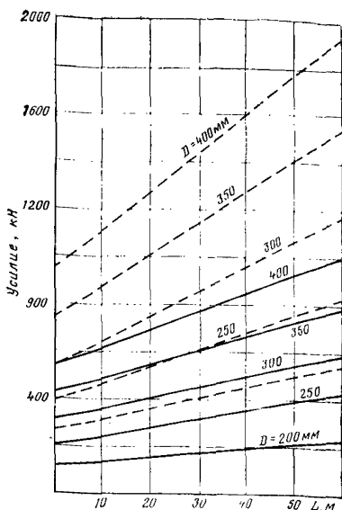
Рис. 49. График для определения усилий при прокладке футляров прокальванием (пунктирная линия — для песчаных грунтов, сплошная — для глинистых)
