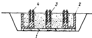
Рис. 22. Сборно-монолитный фундамент под оборудование
