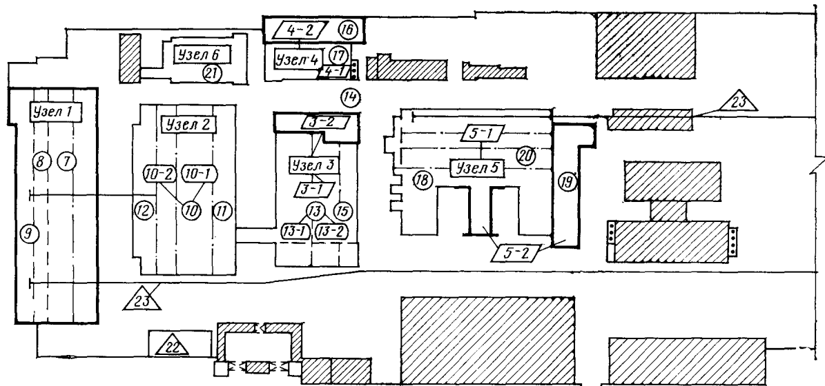
Рис. 5. Схематический план реконструируемого станкостроительного завода с разбивкой комплекса на узлы
