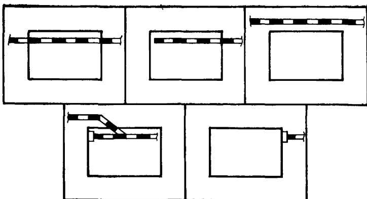
Рис. 30. Возможные варианты прокладки подъездных железнодорожных путей при реконструкции пролетов
