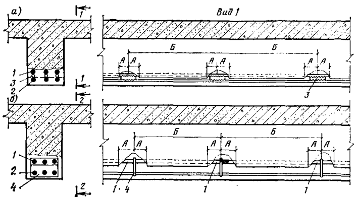
Рис. 41. Усиление балок и ригелей с помощью
