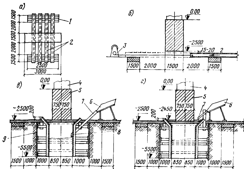
Рис. 16. Вывешивание фундамента под оборудование. Производство работ
