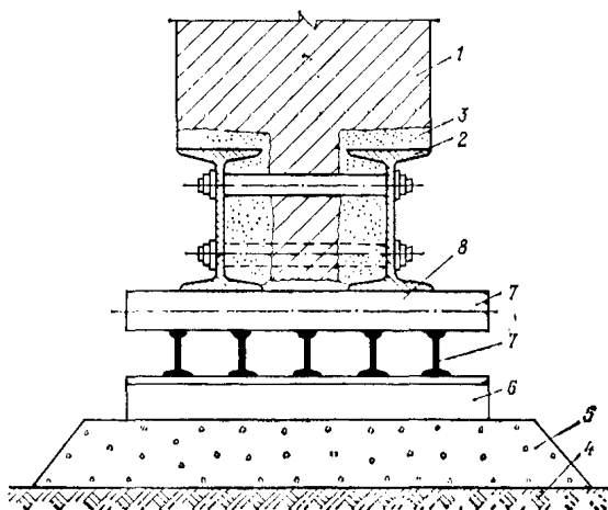
Рис. 7. Схема опирания передвижного здания на рандбалки и устройства путей
