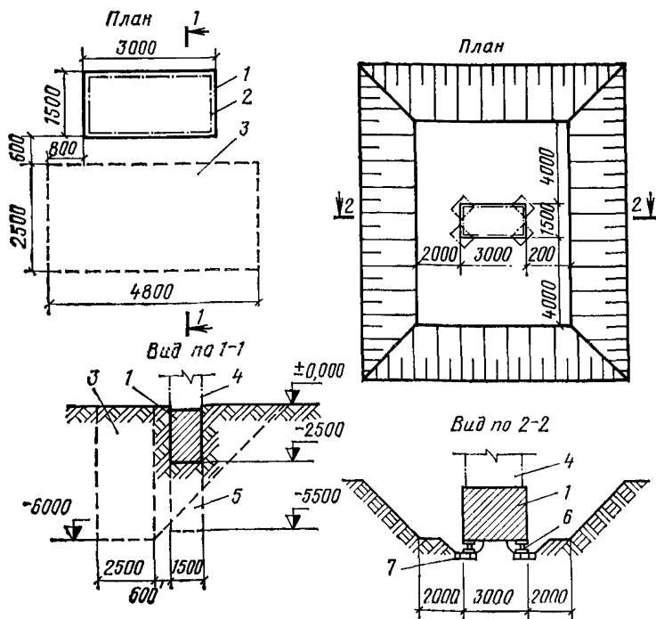
Рис. 15. Вывешивание фундамента под оборудование. Общий вид
