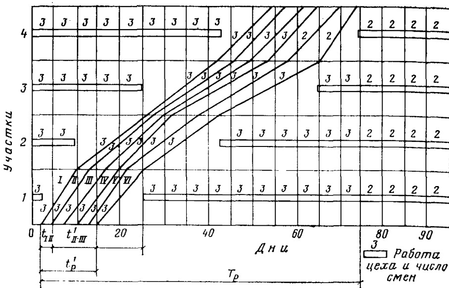
Рис. 2. График потока при реконструкции цеха с частичной остановкой производства (поочередная остановка производства на реконструируемых участках). Цифры 2, 3 означают количество смен работы производства и на строительно-монтажных работах
