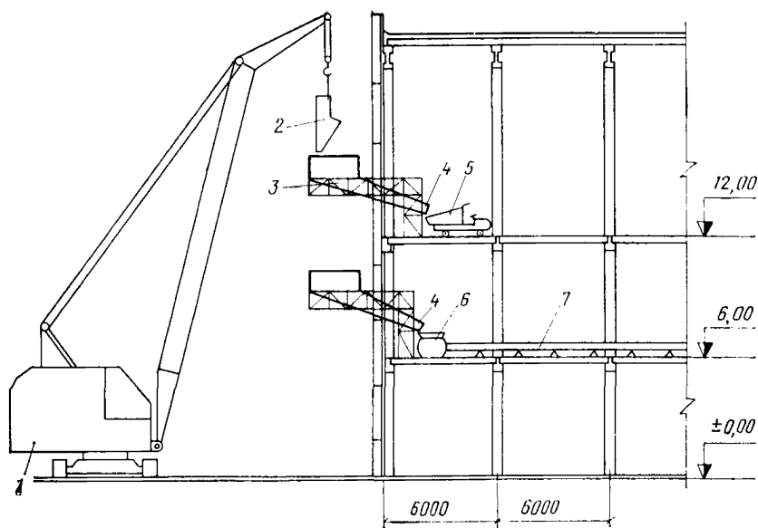
Рис. 21. Подача бетонной смеси при выполнении работ в многоэтажном здании
