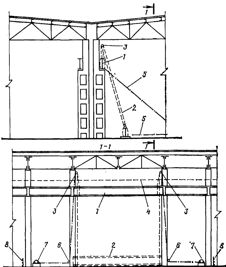
Рис. 24. Замена подкрановых балок лебедками
