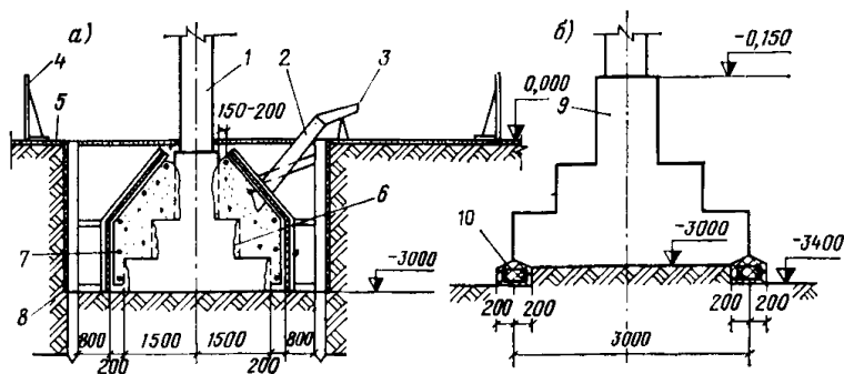
Рис. 39. Уширение фундаментов колонн
