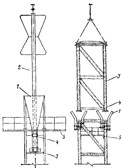
Рис. 38. Схема приспособлений типа «ловушка» для вертолетного монтажа
