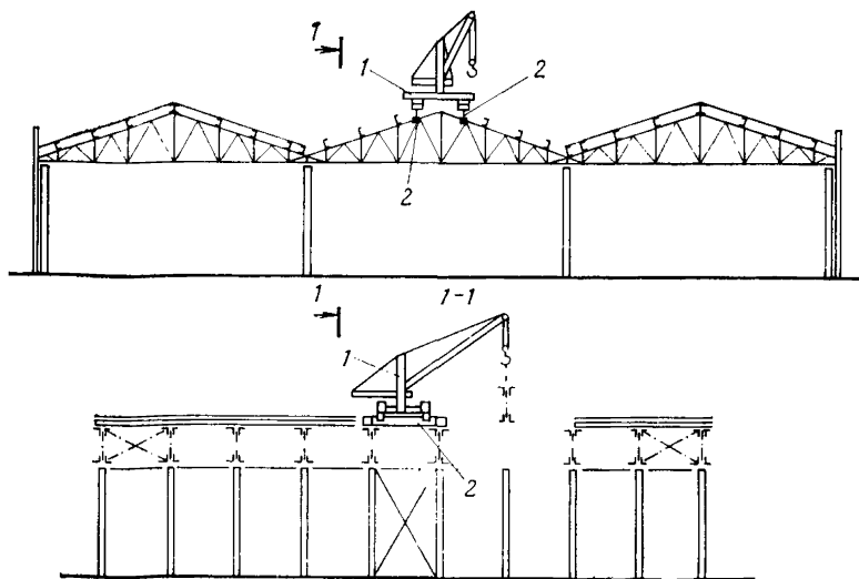
Рис. 23. Замена конструкций покрытия с помощью крышевого крана 1 — крышевой кран; 2 — ездовые балки
