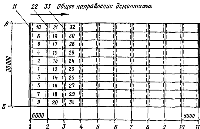
Рис. 10. Пример последовательности демонтажа покрытия цеха
