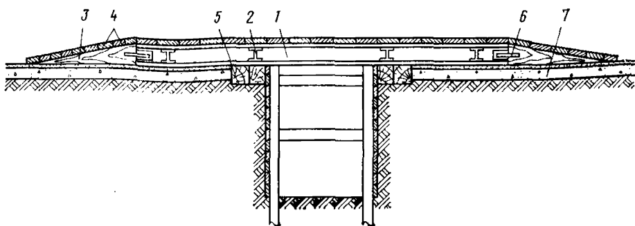
Рис. 45. Временный мост для автомобильной дороги
