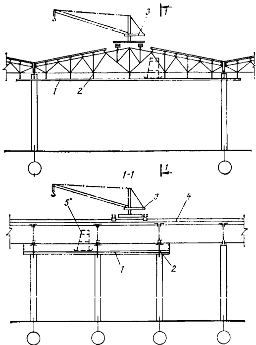
Рис. 33. Подвесной рабочий настил при усилении кровли
