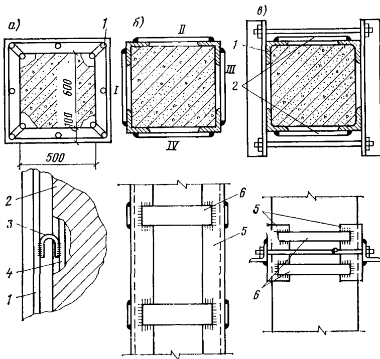
Рис. 40. Усиление колонн обоймами
