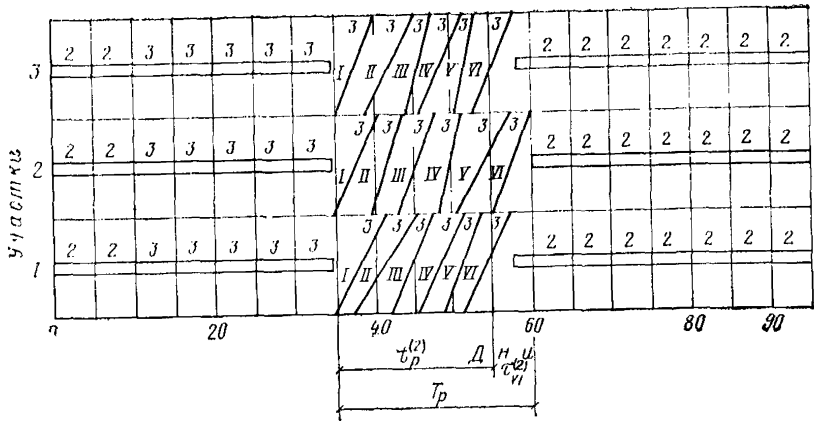
Рис. 4. График потока при реконструкции цеха с полной остановкой производства на период реконструкции
