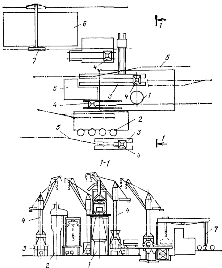
Рис. 37. Эстакадный способ монтажа доменной печи
