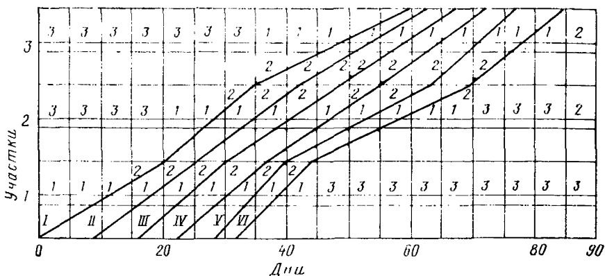
Рис. 3. График потока при реконструкции цеха с частичной остановкой производства (уменьшение числа смен работы в период реконструкции участков цеха)
