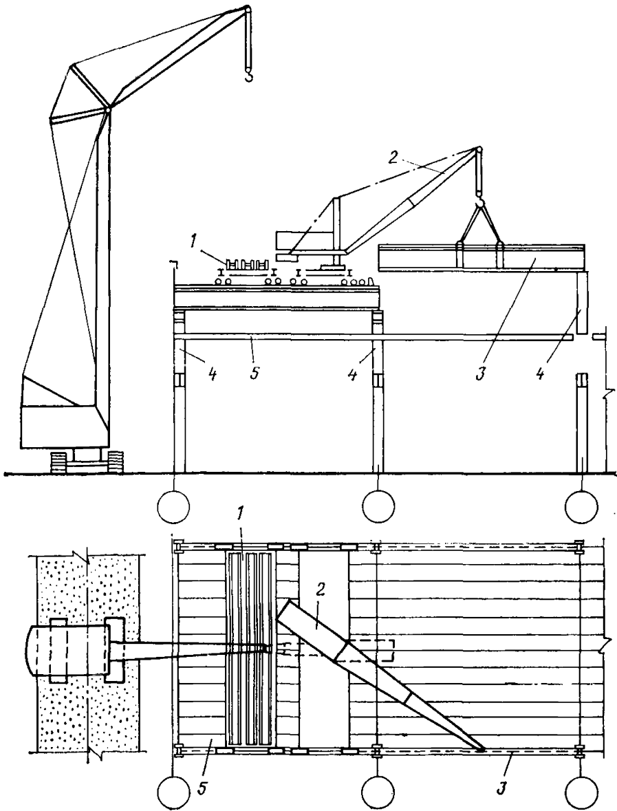
Рис. 32. Схема монтажа колонн и балок с рельсами
