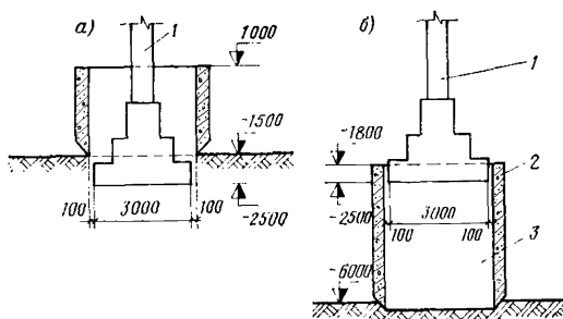
Рис. 17. Устройство железобетонной рубашки у фундаментов колонны
