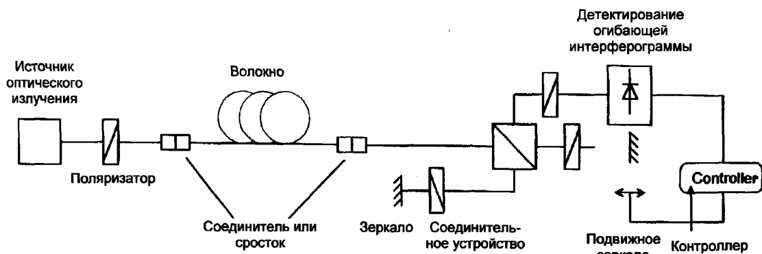
С.2а – интерферометр Мичельсона
