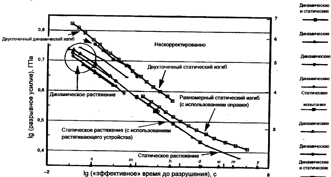
Рисунок Н.1 – Результирующие графики зависимости предела прочности при разрыве от времени при проведении испытаний по круговой системе
