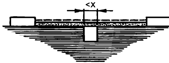
Рисунок G.2 – Расстояние утечки между подвижными и неподвижными контактодержателями из изоляционного материала
