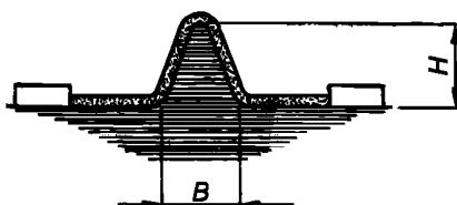
Рисунок G.1 – Размеры ребер
