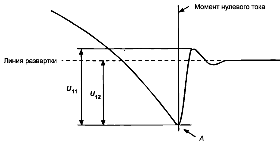
Рисунок Е.1 – Определение фактического значения коэффициента \gamma
