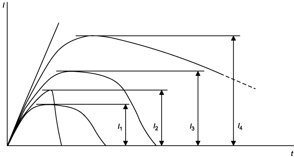
I_1 – первая калибровка; I_2 – фактический ток отключения; I_3 – вторая калибровка; I_4 – отключающая способность Рисунок 15 – Определение ожидаемого тока отключения после проведения первой калибровки при токе, меньшем номинальной отключающей способности [см. 8.3.4.1.8, перечисление b)]
