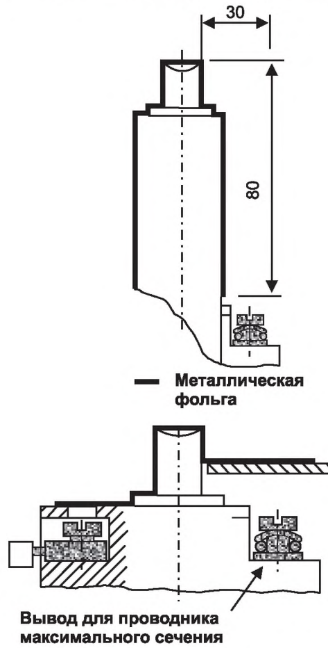
Рисунок R.2 – Оперативное пространство для нажимной кнопки
