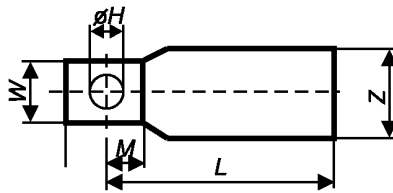
Рисунок Р.1 – Размеры
