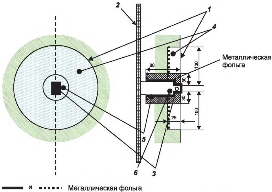
Рисунок R.2 – Оперативное пространство для нажимной кнопки
