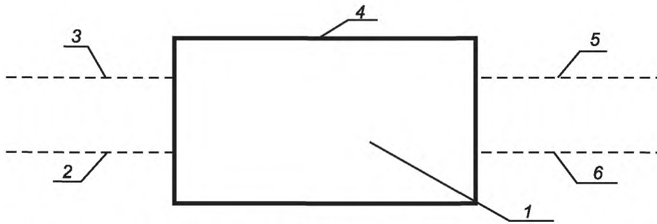
1 – оборудование/аппаратура; 2 – порт функционального заземления; 3 – вывод сигнальной цепи; 4 – оболочка порта; 5 – вывод питания (цепи управления); 6 – вывод главной цепи Рисунок 17 – Пример порта
