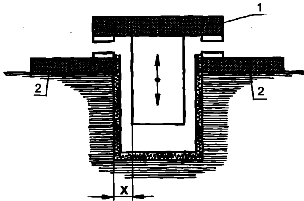
1 – подвижный контактный мостик; 2 – неподвижные контакты;
