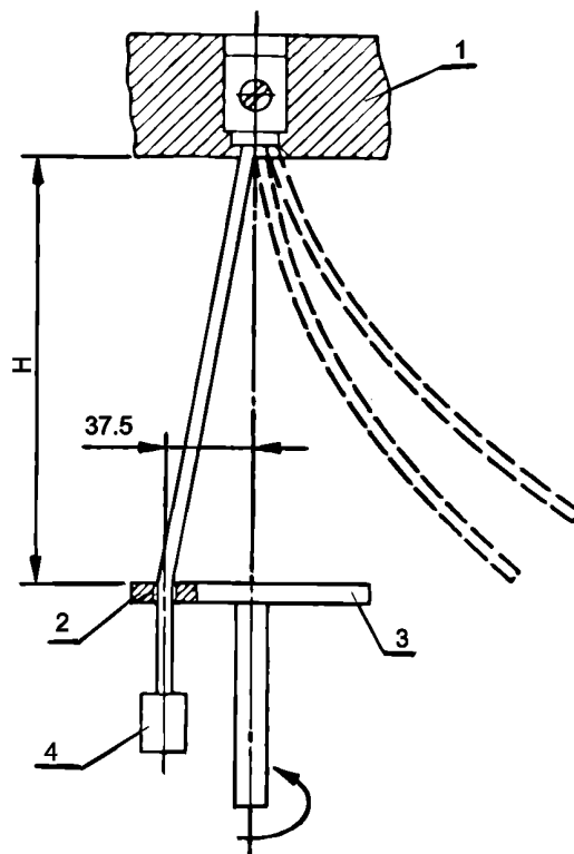
1 – узел фиксации; 2 – гильза; 3 – диск; 4 – груз
