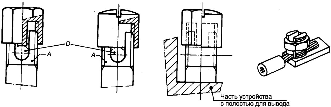
A – неподвижная часть; D – место для проводника.
