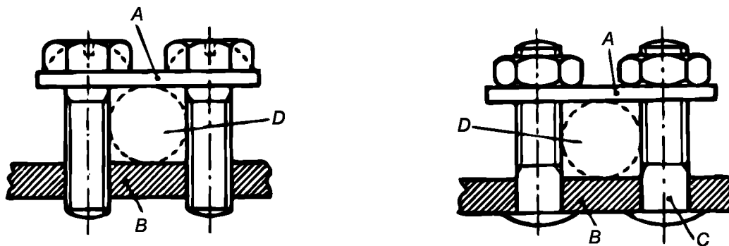
Рисунок D.3 – Штифтовые зажимы
