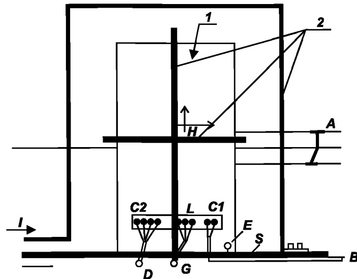
1 – испытуемый аппарат (ИА); 2 – катушка индуктивности; А – заземление безопасности; В – к источнику питания; С1 – цепь источника питания; С2 – сигнальная цепь; D – имитатор источника сигналов; E – вывод заземления; G – к испытательному генератору; H – сила электромагнитного поля; I – индукционный ток; L – линия связи; S – изоляционная опора Рисунок 23 – Испытательная установка для проверки на устойчивость к электромагнитным полям промышленной частоты
