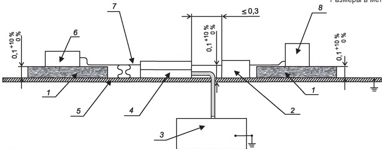
Рисунок 21 – Испытательная установка для проверки на устойчивость к кондуктивным электромагнитным помехам, наведенным на силовые линии радиочастотными электромагнитными полями
