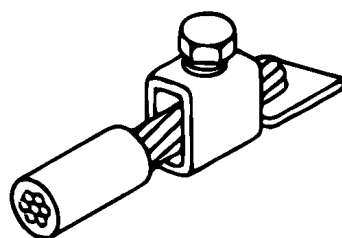
Выводы с прокладкой
