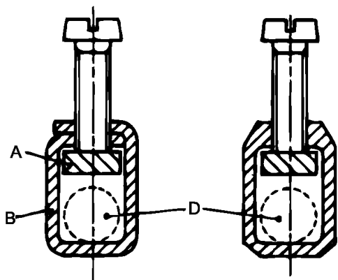
Выводы с непрямой передачей давления
