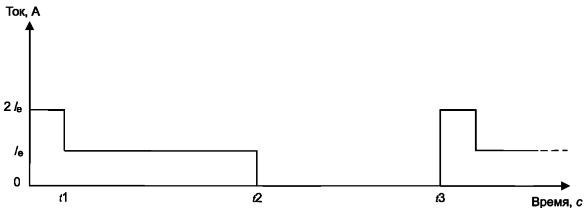
Рисунок S.4 – Временные интервалы коммутационного переключения для цифровых выходов постоянного тока
