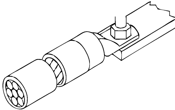
A – запорное устройство; B – кабельный наконечник или шина; F – неподвижная часть; E – штифт Зажим под наконечник – резьбовой или штифтовой зажим предназначен для зажима кабельного наконечника или шины с помощью винта или гайки.
