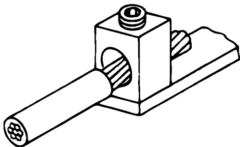
Выводы с прямой передачей давления
