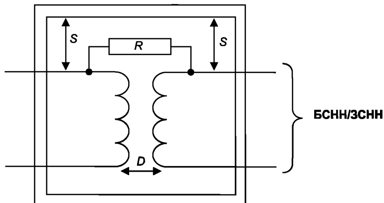
Рисунок N.1 – Пример подсоединения компонента между разделенными цепями
