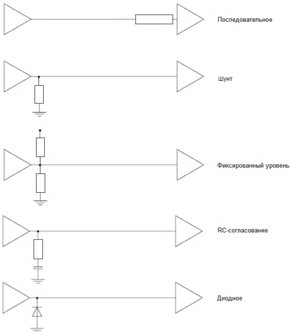
Рисунок 3 – Согласование нагрузок
