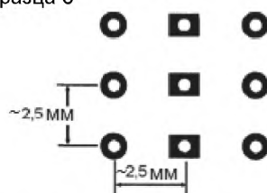
Единичный тест-купон волнового сопротивления Схема образца 3
