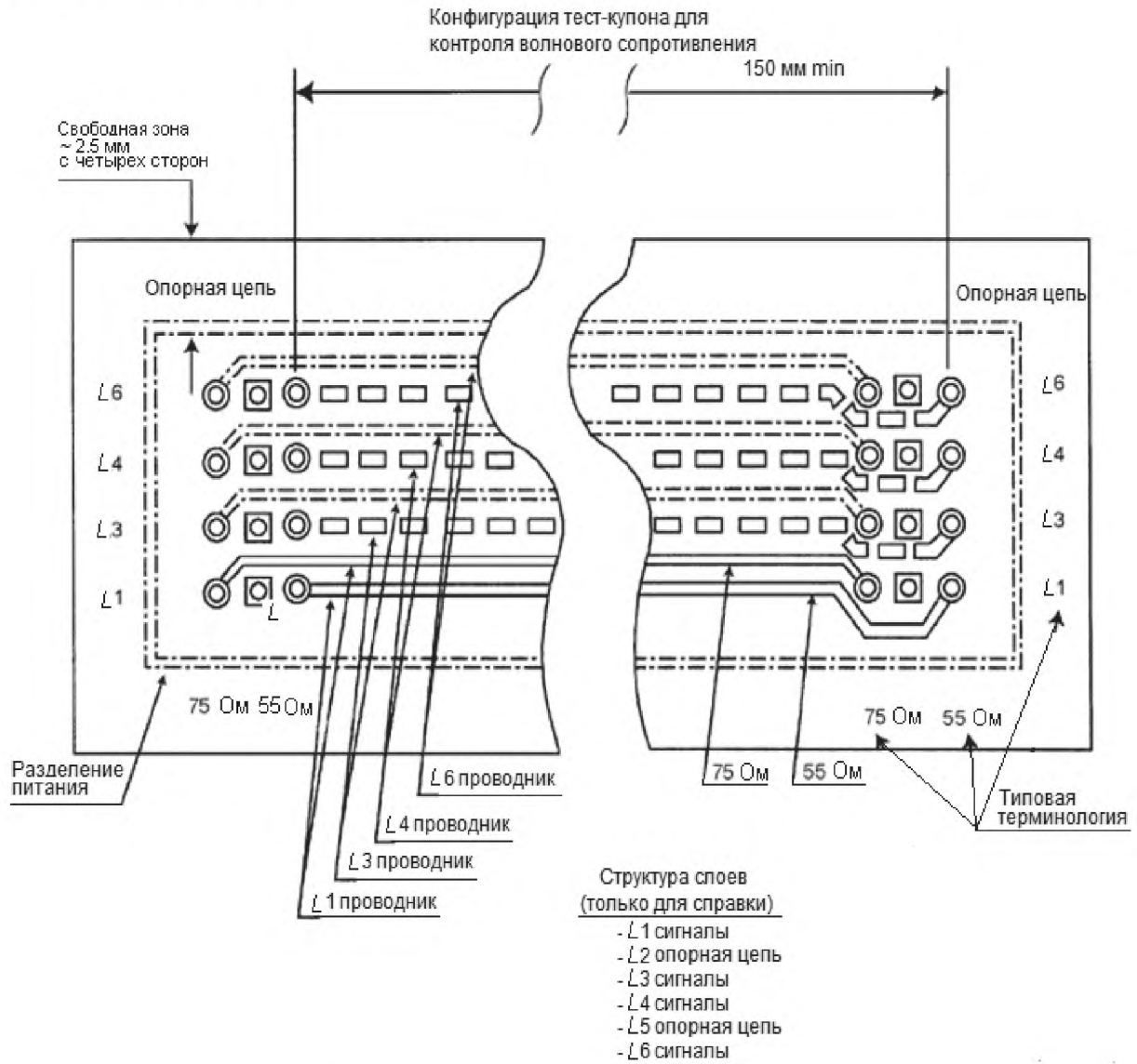
Рисунок 10 – Тест-купон контролируемого волнового сопротивления
