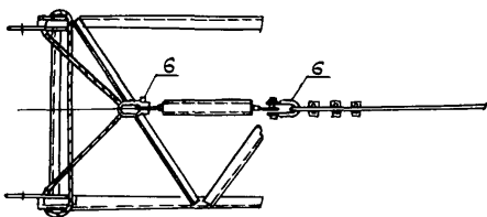
Рис. 1-2 Раскрепление ригельной траверсы временной связью.
