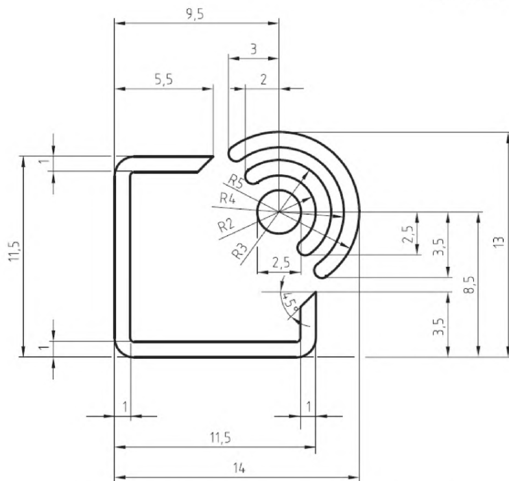
Рисунок В.1 – Структура основы эмблемы радиочастотной идентификации
