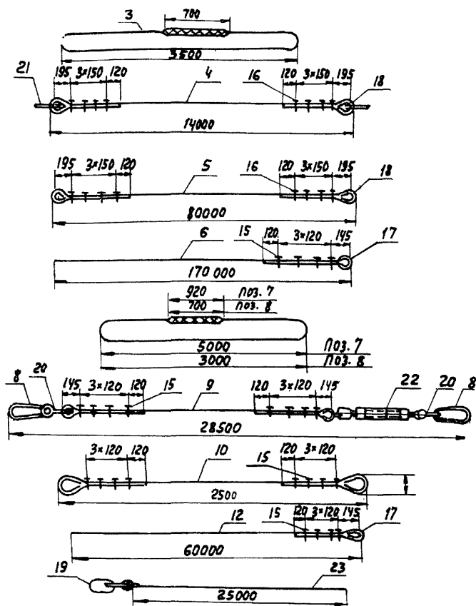
Рис. 5-2. Детали строповки опор ПБ-500-2; ПБ-500-3 (кран К-255)
