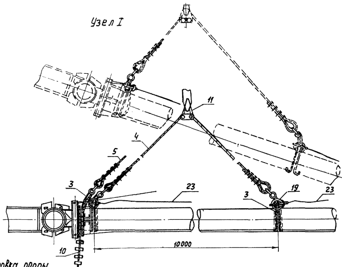
Рис. 5-3. Стрповка опоры
