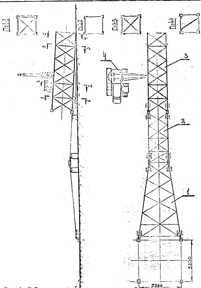
Рис. 13 Сборка 3 ей секции ствола опоры УЭЭО-2.
