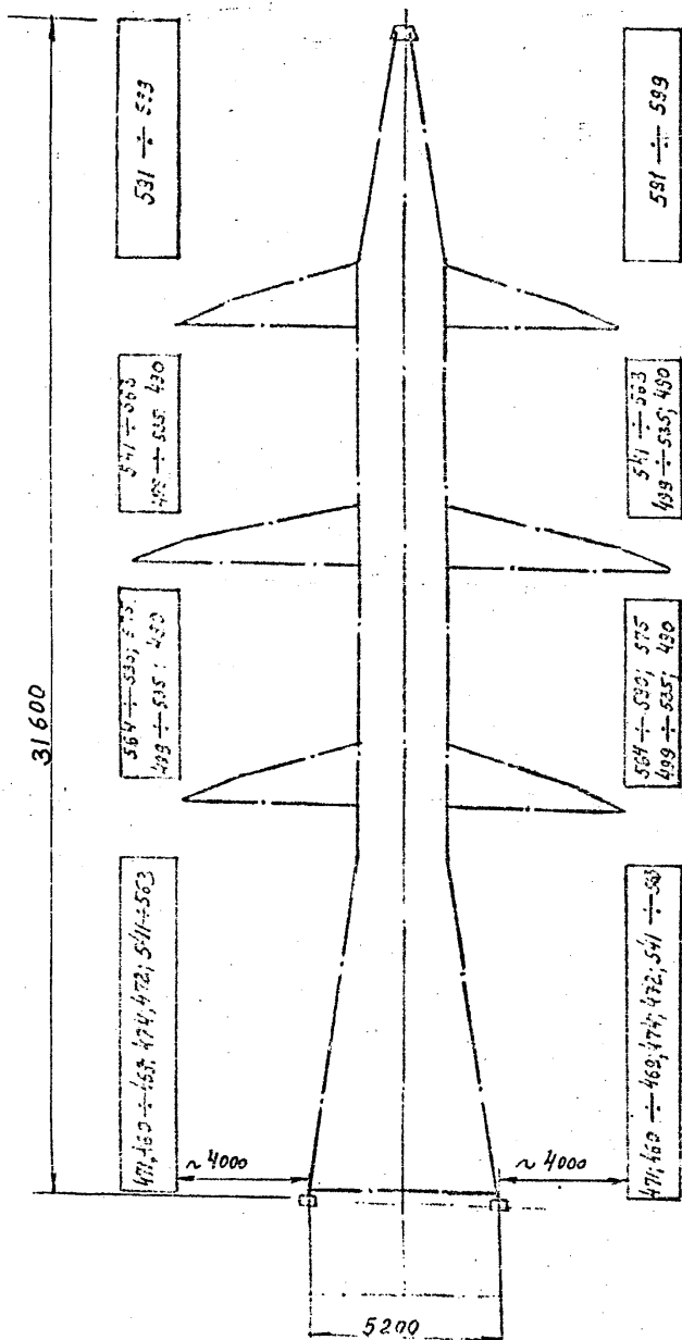
Рис. 11. Раскладка пакетов в деталях опоры 3220-2 на пикете.
