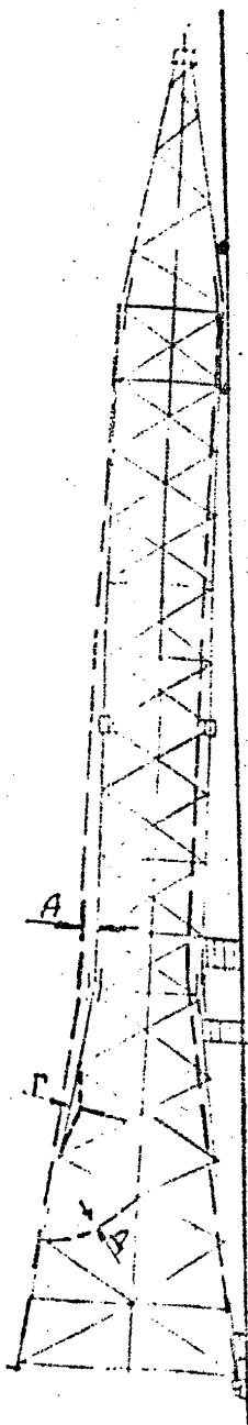
Рис. 47 Допускаемые отклонения при сборке опоры УЭ20-2
