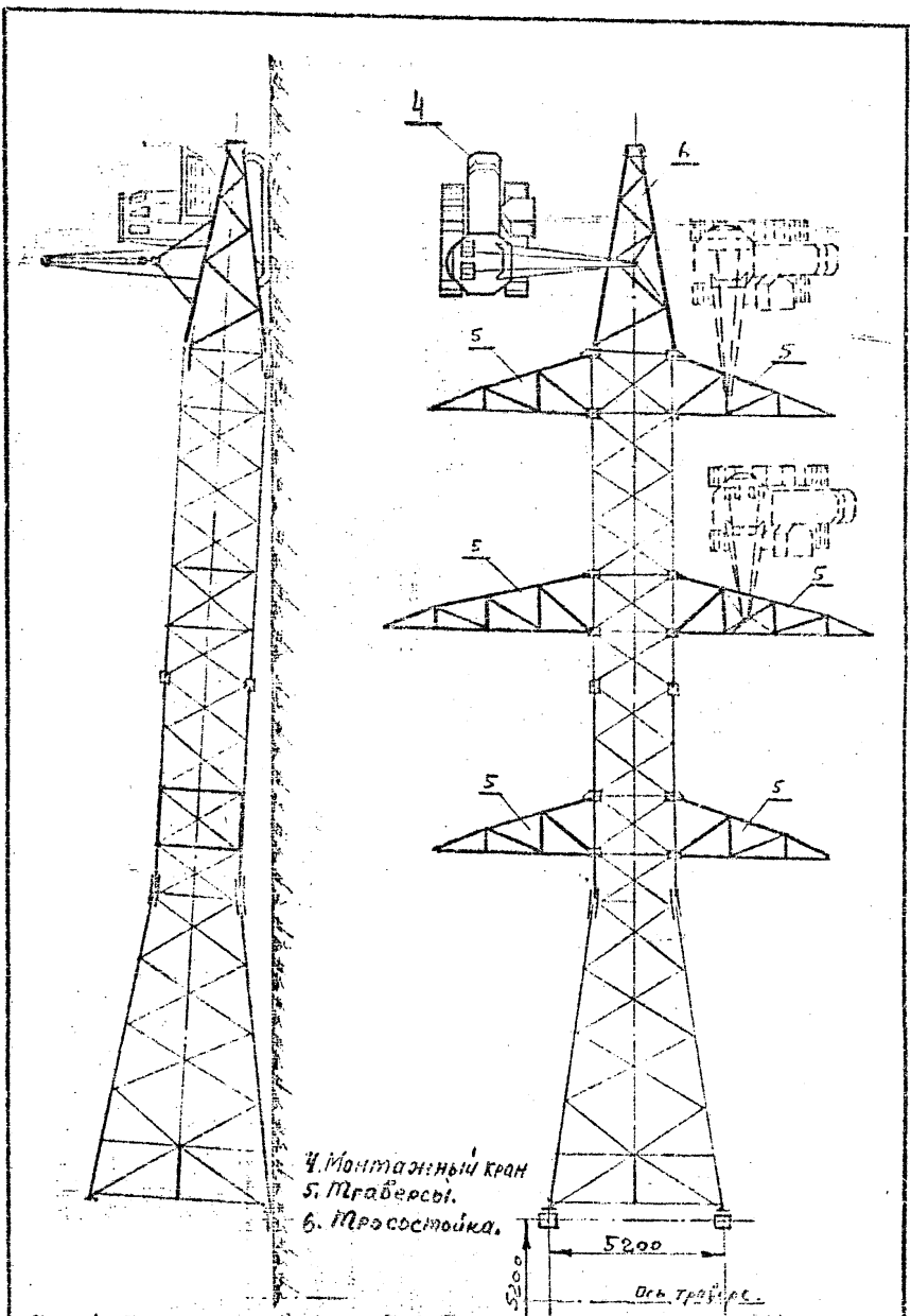
Рис. 46 Пристыковка тросов и тросовый к стволу пром. 4220-2
