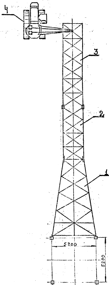
Рис. 42 Сборка нижней плоскости 1 ой 2 ой 3 ей секции опоры УЗ20-2
