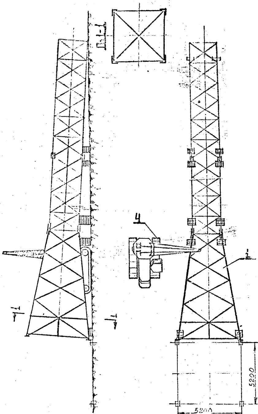
Рис. 15 Сборка 1 ой секции ствбл. опоры 4220-2.
