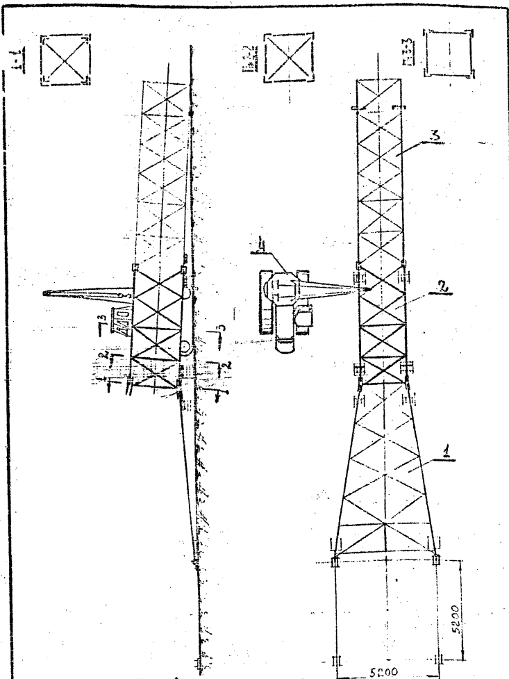
Рис. 44 Сборка 2 ой секции ствблa опоры У220-2.
