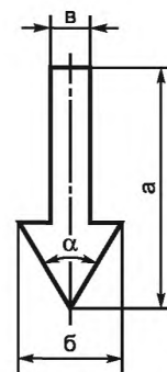
a = 180\text{--}200 мм; b = 80\text{--}100 мм; v = 30\text{--}40 мм; \alpha = 60^\circ\text{--}70^\circ
