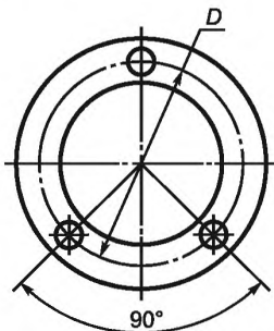
Рисунок 1 — Схема расположения отверстий на посадочной поверхности ССС мачтового, карликового и заградительного мачтового светофора
