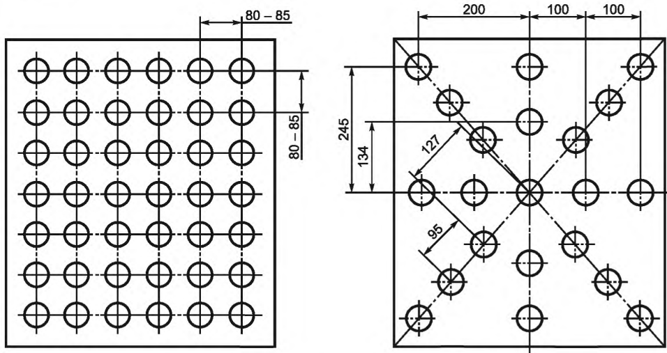
а) указатель буквенный или цифровой б) указатель положения
