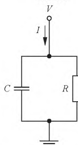
Рисунок 3 – Эквивалентная электрическая цепь заряжения проводника
