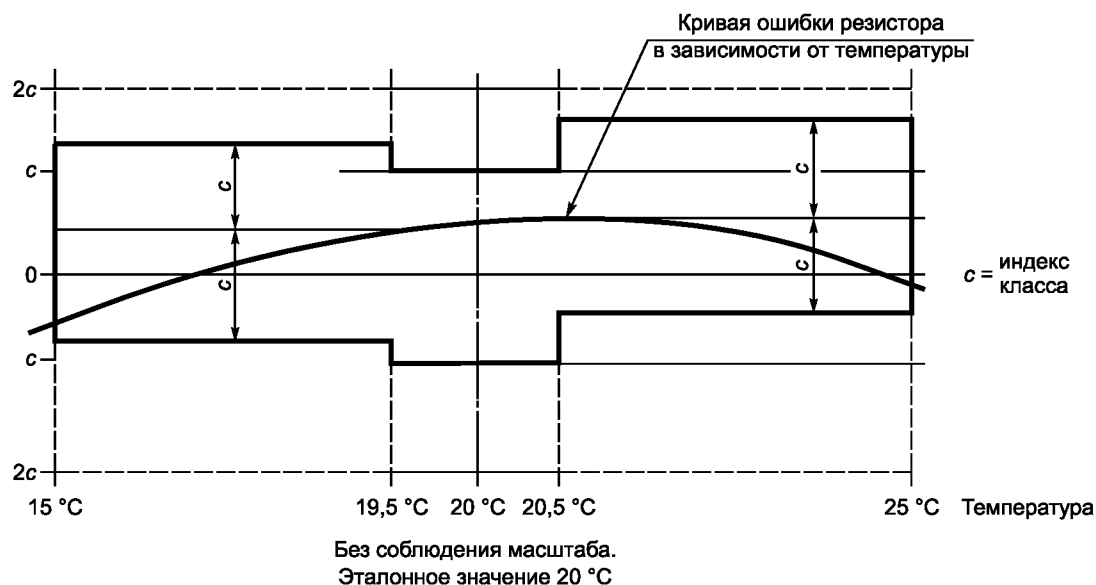
Рисунок 1 — Влияние температуры
