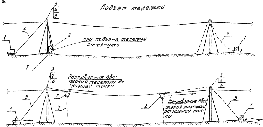
Рис. 4-1. Установка дистанционных распорок на грозозащитном тресе;
