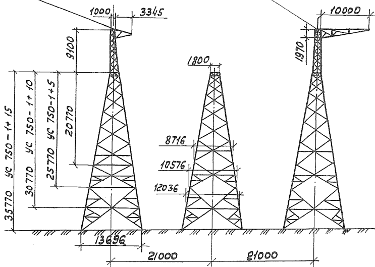
Рис. 0-6. Якорно-узловые опоры типа УС-750-1; УС 750-1+5; УС 750-1+10; УС 750-1+15 (Проект ОДП ЭСП 10224ТМ - 77-1).
