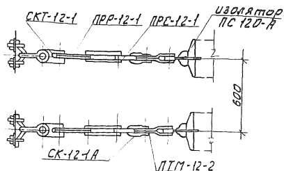
Рис. 0-2. Натяжное двухцепное крепление троса из 8 изоляторов ПС 120-А. Масса гирлянды 133,1 кг. (ЭСП ОДП черт. № 8594-26-87е)
