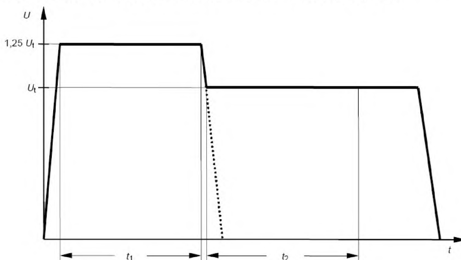
Рисунок 1 – Испытательное напряжение
