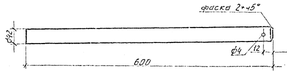
Такелажная деталь
