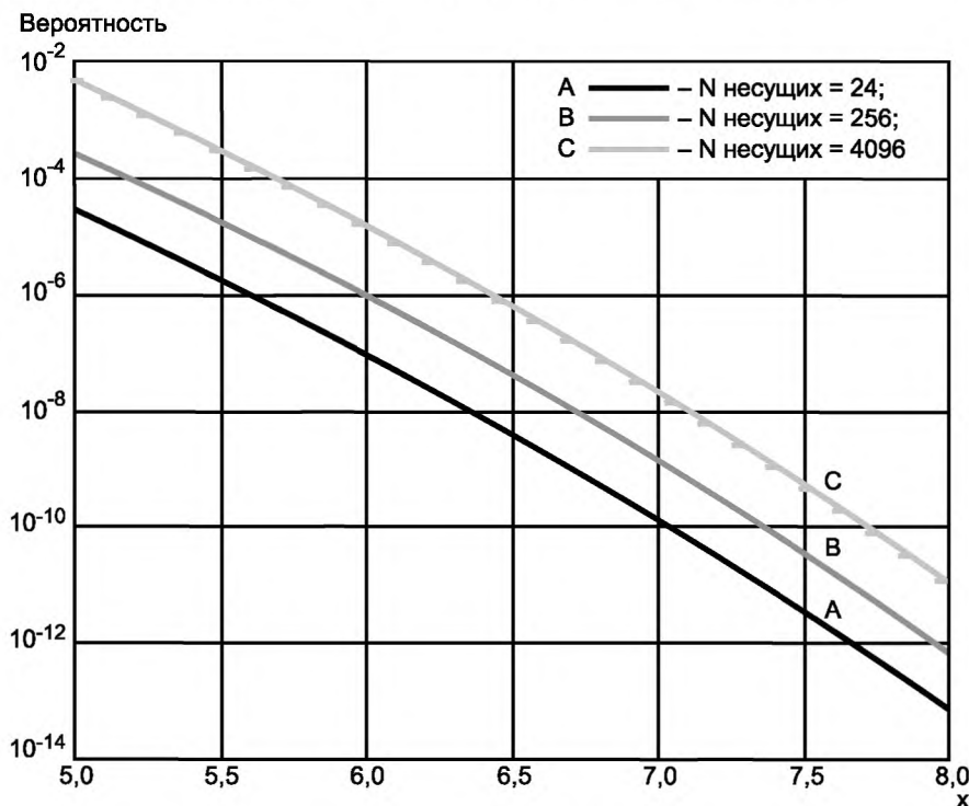
Рисунок А.3 — Вероятность символа с CF > x
