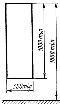
Черт. 1
