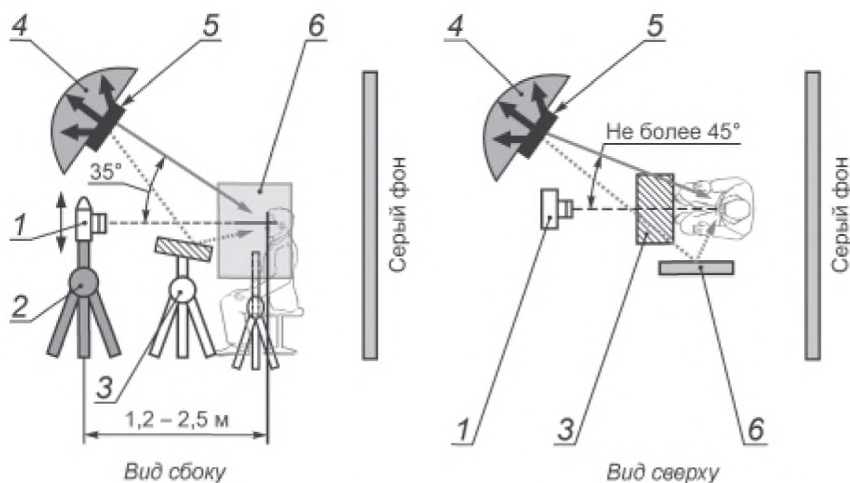
1 — камера; 2 — штатив; 3 — отражающая панель; 4 — ламповый отражатель; 5 — источник освещения; 6 — боковая отражающая панель
