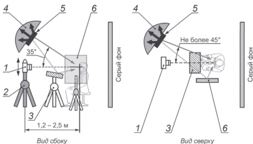
1 — камера; 2 — штатив; 3 — отражающая панель; 4 — ламповые отражатели; 5 — основной источник освещения; 6 — фронтальный источник освещения; 7 — осветитель фона
