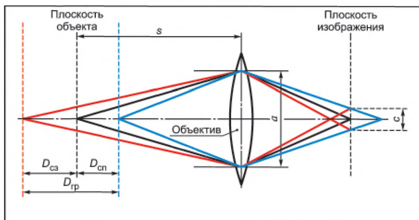
Рисунок С.1 — Параметры для вычисления глубины поля
