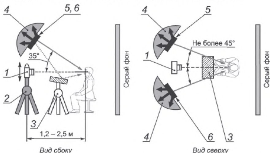
1 — камера; 2 — штатив; 3 — отражающая панель; 4 — ламповые отражатели; 5 — основной источник освещения; 6 — фронтальный источник освещения
