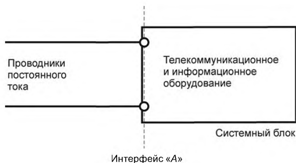
Рисунок 1 — Идентификация интерфейса «А»
