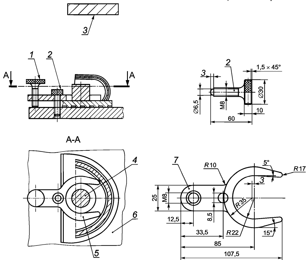
1 — регулировочный винт; 2 — зажимной винт; 3 — ударный боек; 4 — цилиндр из глины для моделирования; 5 — стабилизирующая вилка; 6 — опорная плита; 7 — толщина = 10 мм
