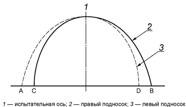
Рисунок 2 — Определение испытательной оси
