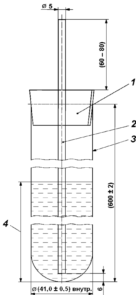
Рисунок 1 – Окислительная ячейка
