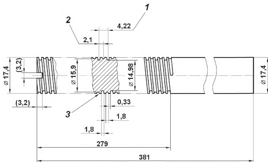
1 – ход; 2 – шаг; 3 – двухходовая резьба Материал – бронза.
