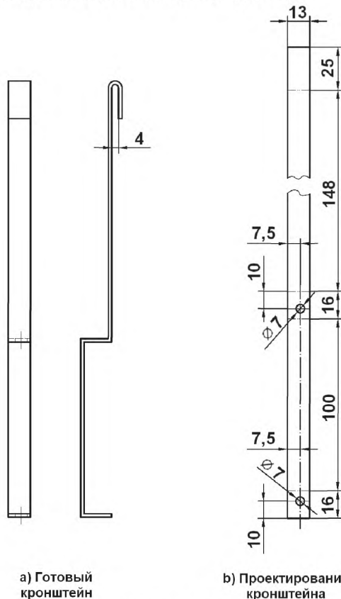
Рисунок 2 – Держатель для термометра
