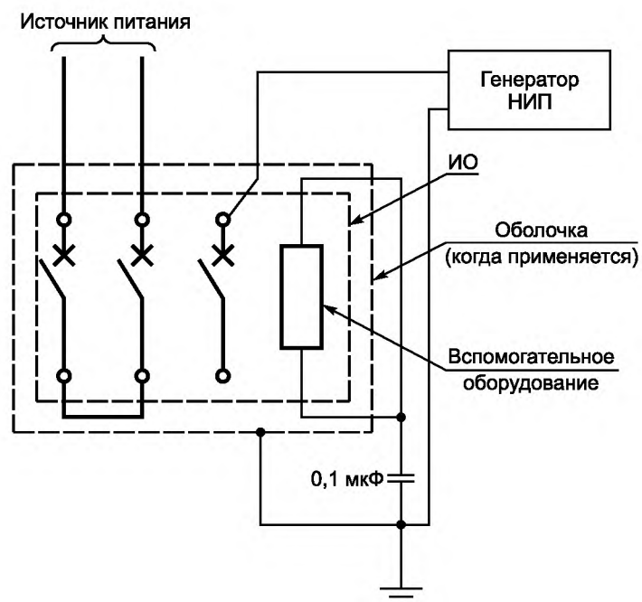
Рисунок 13 — Цепь для испытаний на устойчивость к наносекундным импульсным помехам (НИП). Двухфазная конфигурация с последовательным подключением полюсов
