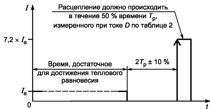
Рисунок 26 — Испытание тепловой памяти
