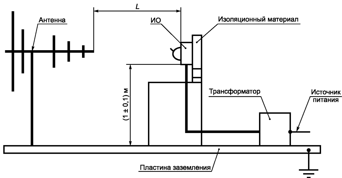
Рисунок 25 — Испытательная установка излучения радиопомех
