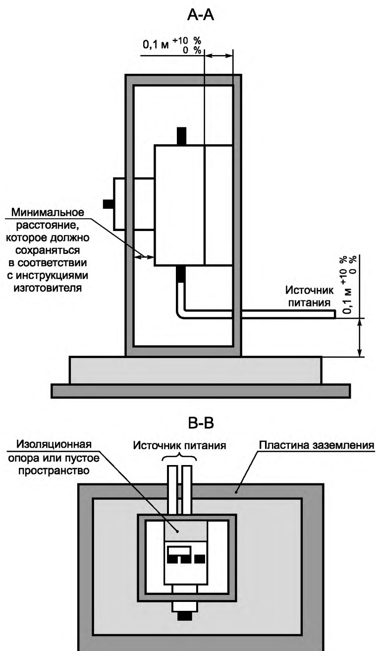
Рисунок 2b — Сечения A-A и B-B
