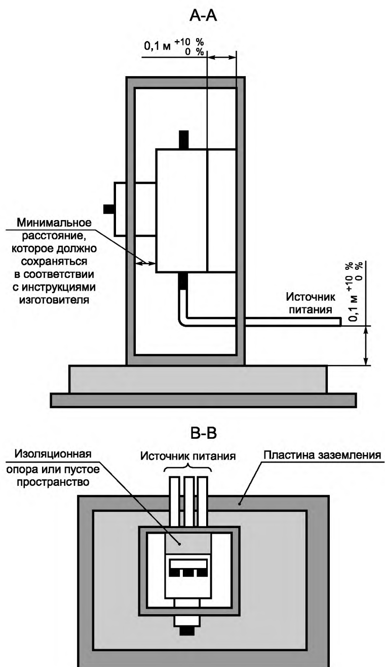
Рисунок 4b — Сечения А-А и В-В
