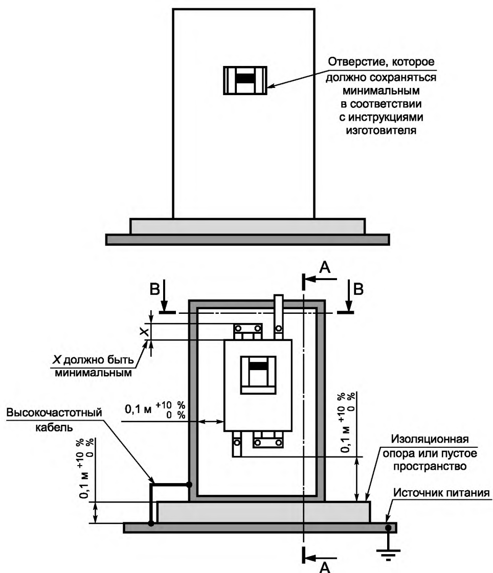
Рисунок 3а — Вид спереди
