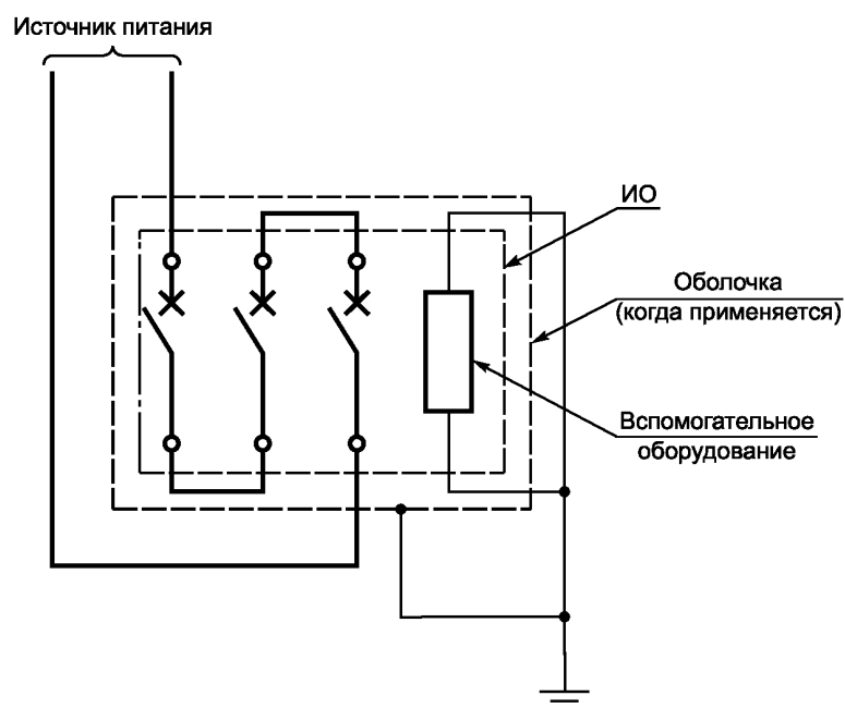
Рисунок 6 — Испытательная цепь для испытаний на излучение помех, устойчивость к гармоническим составляющим, провалам напряжения, электростатическим разрядам и электромагнитным полям. Трёхфазная конфигурация с последовательным подключением полюсов
