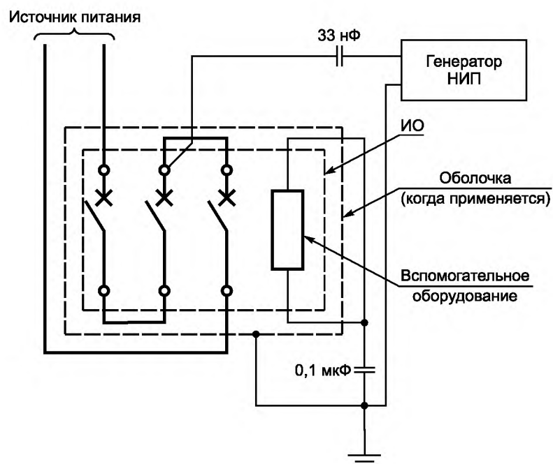
Рисунок 14 — Цепь для испытаний на устойчивость к наносекундным импульсным помехам (НИП). Трехфазная конфигурация с последовательным подключением полюсов
