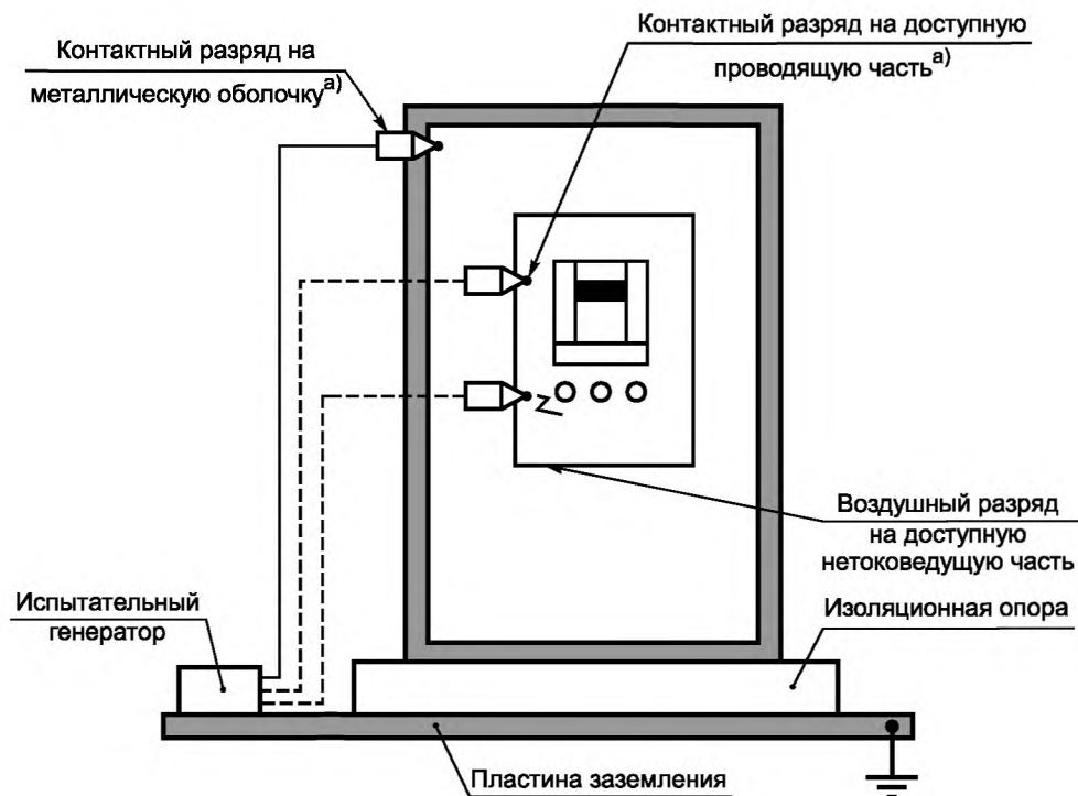
Рисунок 7 — Испытательная цепь для испытаний на излучение помех, устойчивость к гармоническим составляющим, провалам напряжения, электростатическим разрядам и электромагнитным полям. Трёхфазная конфигурация
