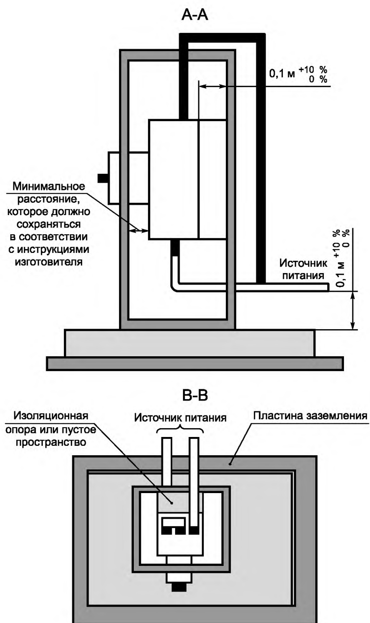
Рисунок 3b — Сечения A-A и B-B
