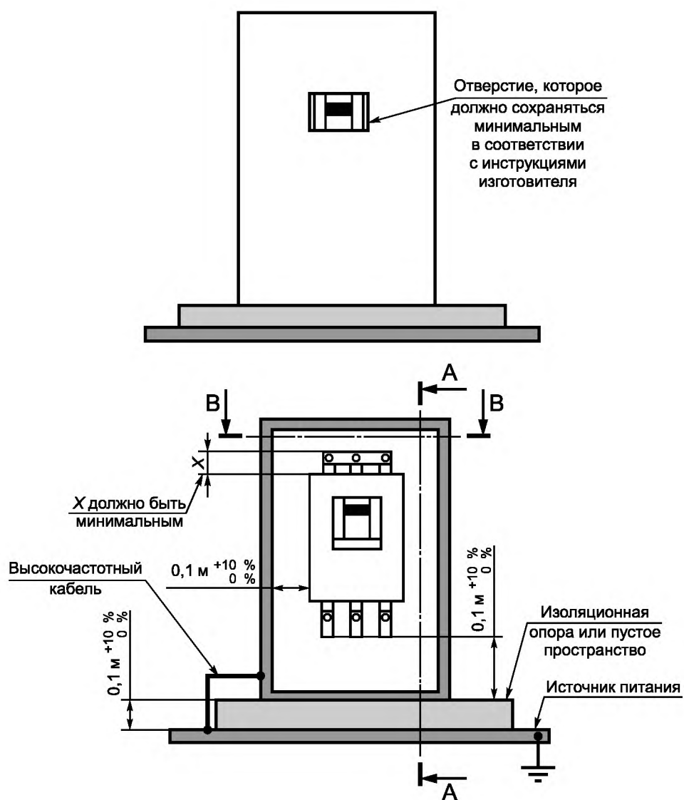
Рисунок 4а — Вид спереди
