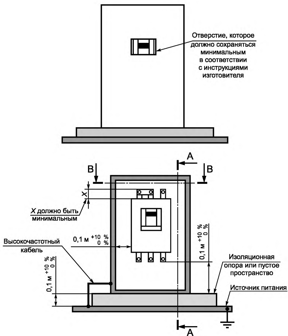
Рисунок 2а — Вид спереди
