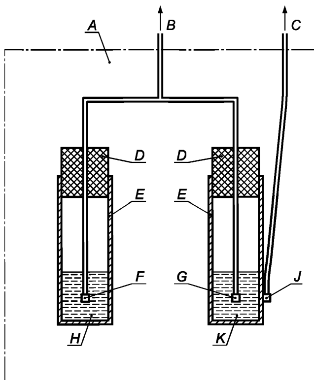
A — печь; B — к милливольтметру ( T_1 - T_2 ); C — к милливольтметру ( T_3 ); D — пробки; E — пробирки; F — термодара № 1 ( T_1 ); G — термодара № 2 ( T_2 ); H — 100 см 3 образца; J — термодара № 3 ( T_3 ); K — 100 см 3 эталонной химической продукции
