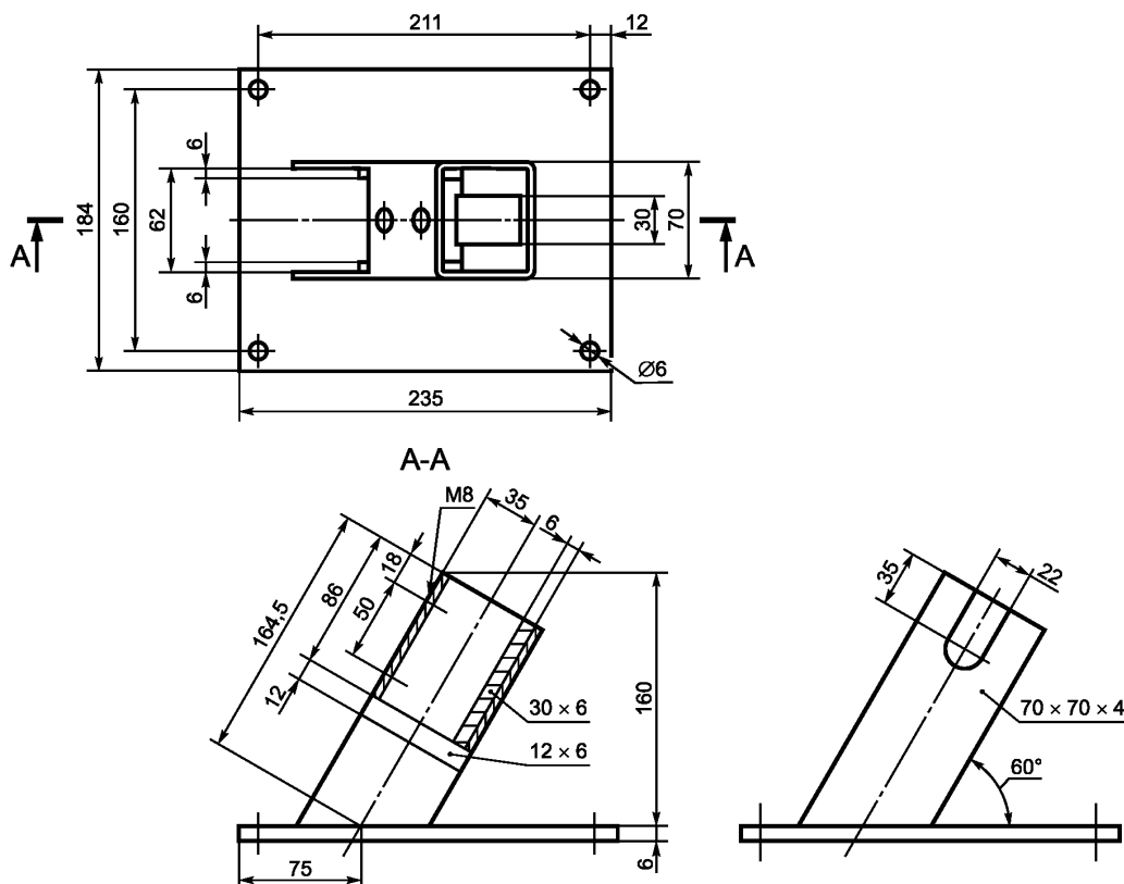
Рисунок 8 — Опорный стэнд
