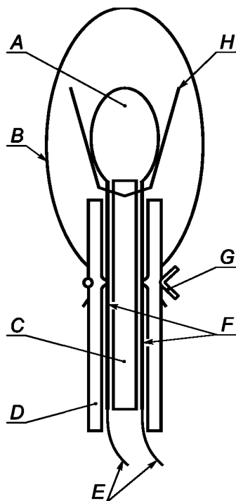
A—мостик накаливания; B—пленка из поливинилхлорида; C—изоляция; D—трубка из кремнийорганического каучука; E — запальные выводы; F — контакты из фольги; G — проволока для водонепроницаемой герметизации; H — запальный кембрик
