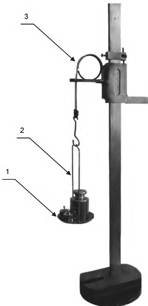
1 – чашка с гирьками; 2 – подвеска; 3 – поршневое кольцо с незамкнутым замком
