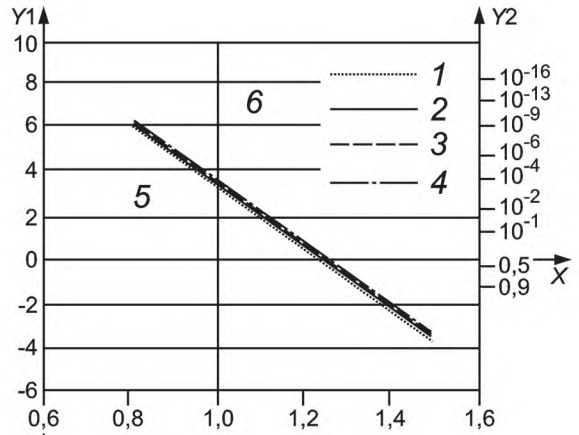
b – Самое глубокое несовершенство для 50 труб, средний запас прочности – 1,3
