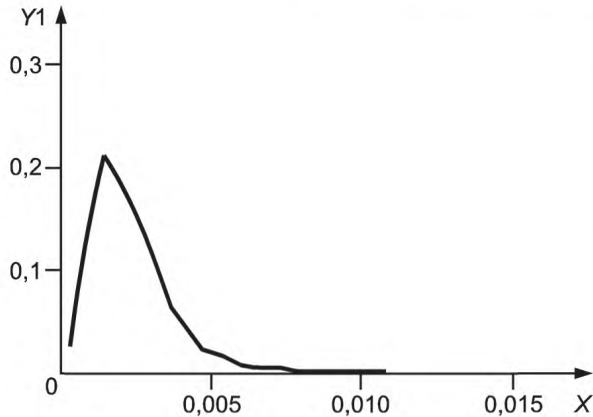
а — Функция распределения вероятностей PDF
