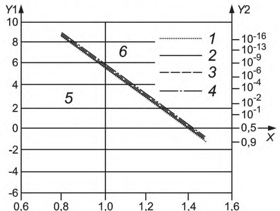
d – Самое глубокое несовершенство для 50 труб, средний запас прочности – 1,5
