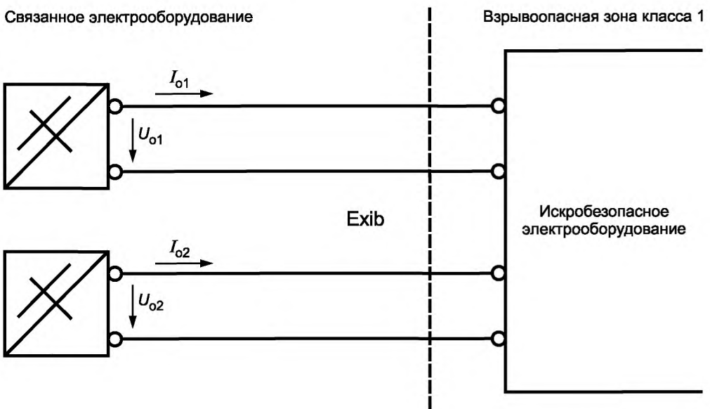
Рисунок I.2 — Параллельное соединение. Суммирование значений тока
