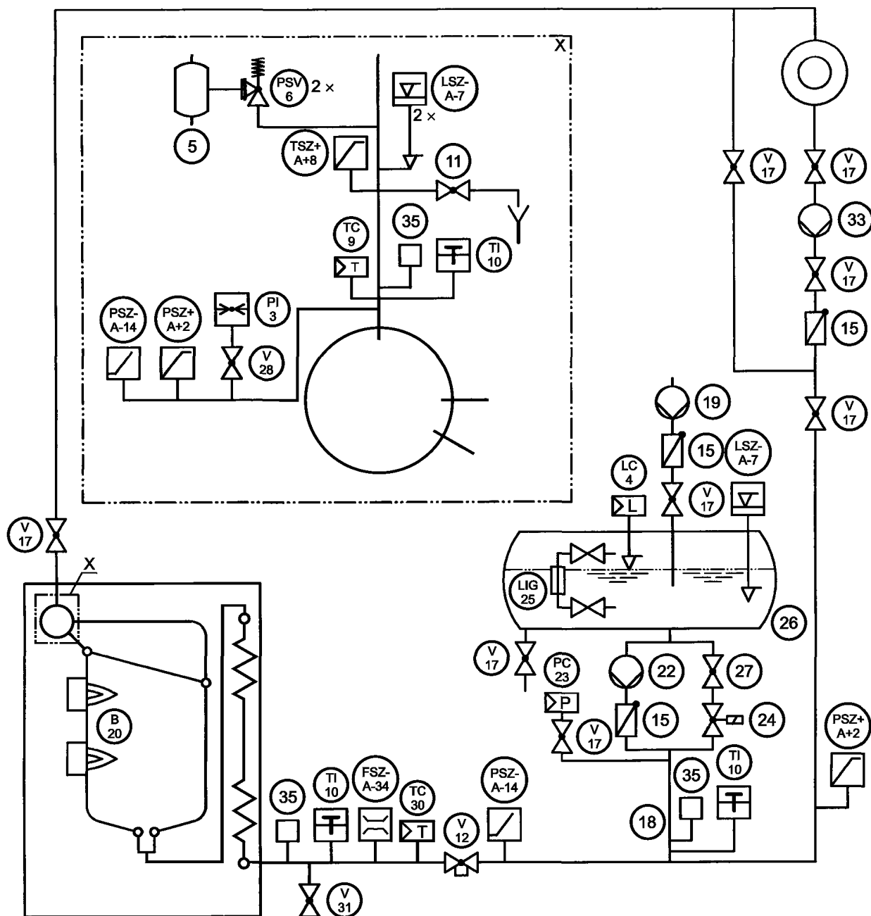
Рисунок В.4-6 — Установки с принудительной циркуляцией, нижней подпиткой воды, насосами поддержанием давления из внешнего источника
