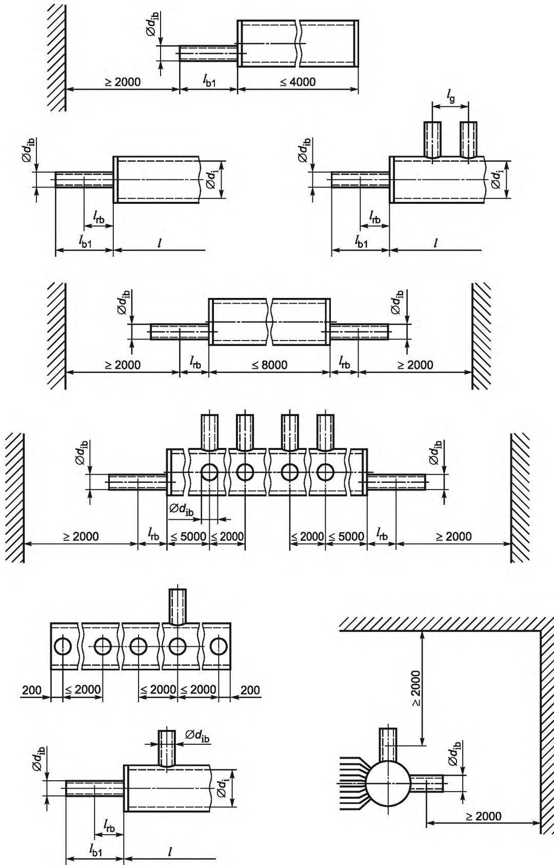
Рисунок 4.6-1 — Примеры расположения отверстий
