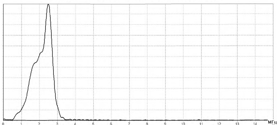
Рисунок 2 – Амплитудный спектр для сильно корродированной резьбы.
