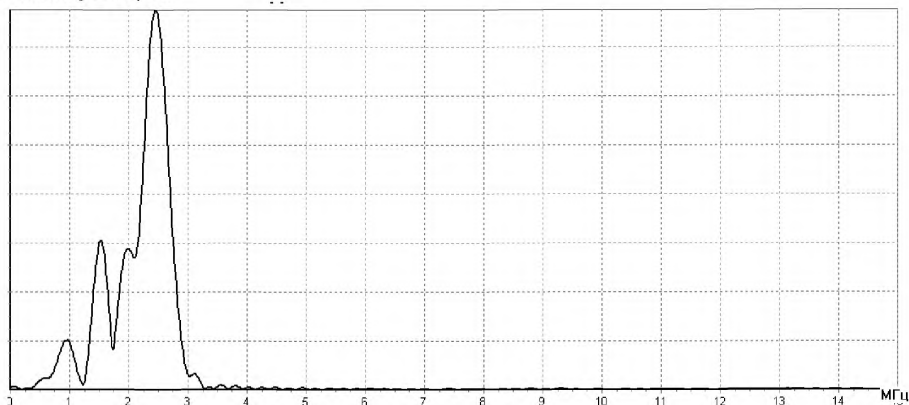
Рисунок 1 – Амплитудный спектр для резьбы СОП.
