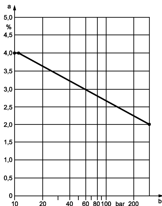
a Максимальные колебания давления. b Давление, p.
