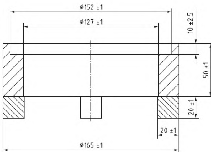
Рисунок А.4 – Вид держателя основы
