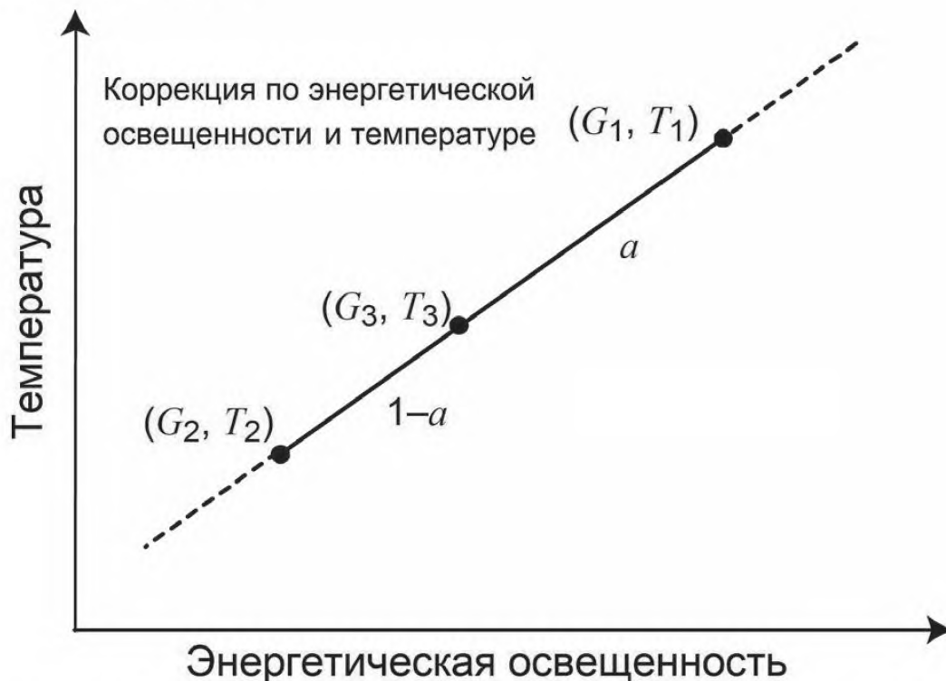
Рисунок 2 – Схематическая диаграмма соотношения значений G_3 и T_3 , которые могут быть выбраны с помощью уравнений (8) и (9) для фиксированных значений T_1 , G_1 , T_2 и G_2 . при коррекции одновременно по энергетической освещенности и температуре. Непрерывная прямая и пунктирная прямая иллюстрируют диапазоны значений, в которых вычисляют G_3 и T_3 путем интерполяции и экстраполяции, соответственно.
