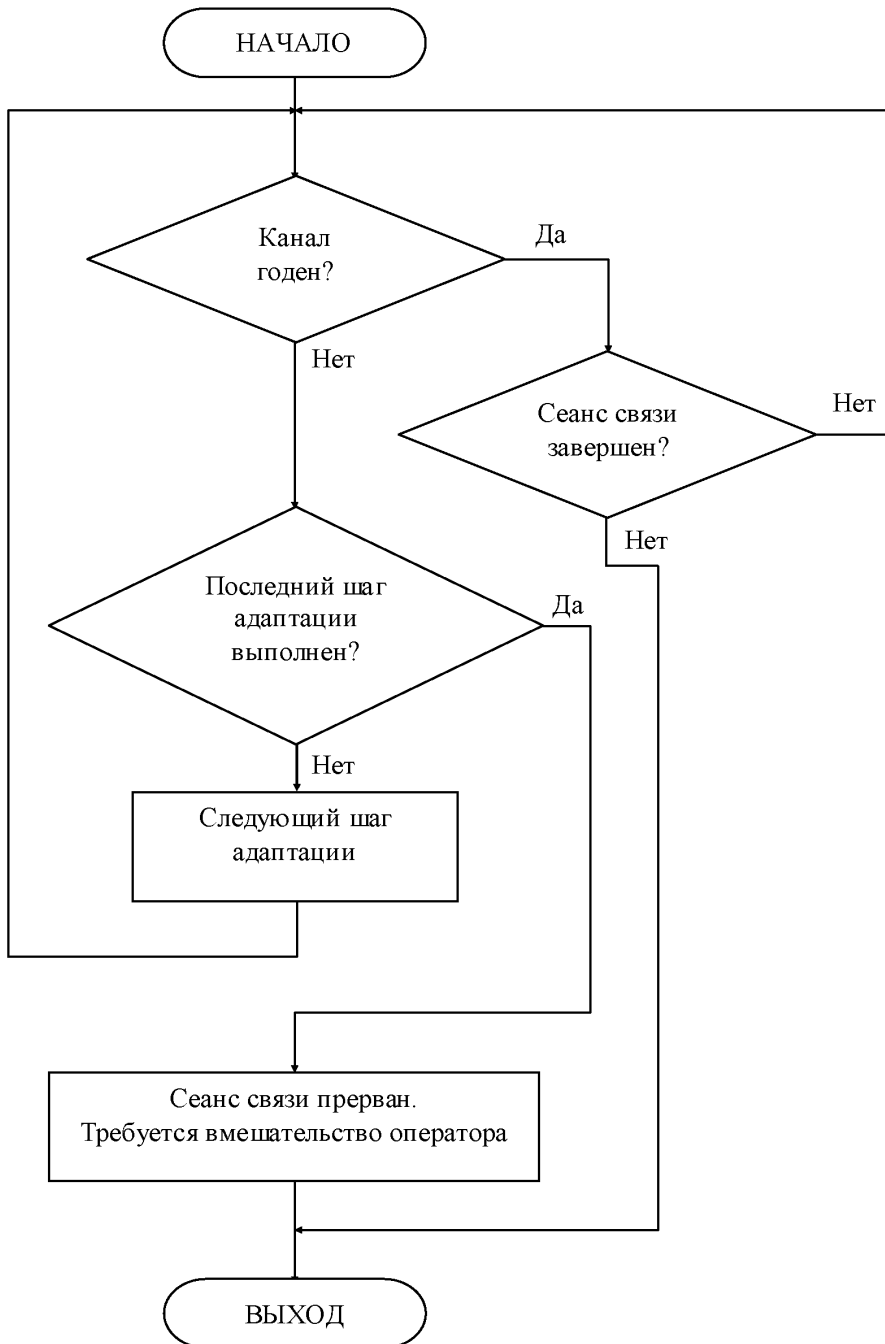
Рисунок 4– Блок-схема алгоритма адаптации
