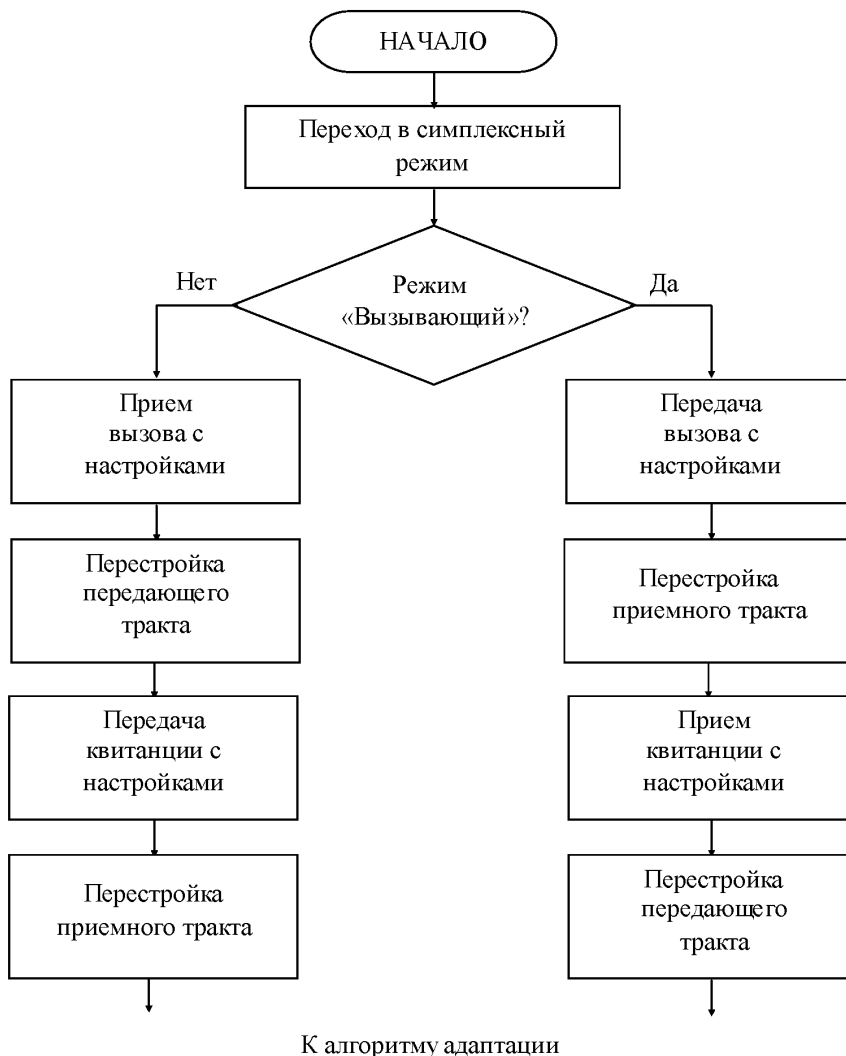
Рисунок 3 – Блок-схема алгоритма перехода в дуплексный режим
