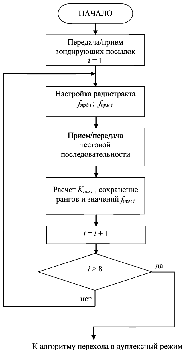
Рисунок 2 – Блок-схема алгоритма ранжирования частот радионаправления
