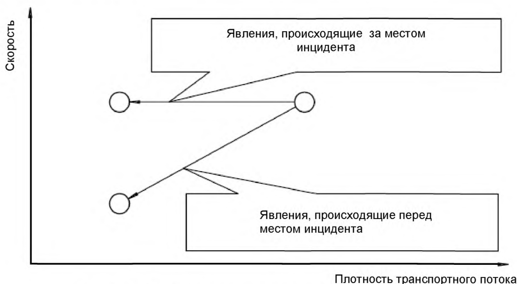
Рисунок 1.2 – Модель явлений, происходящих при транспортном заторе
