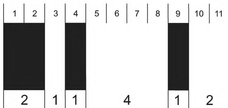
Рисунок 2 — Знак Start A для символа Code 128
