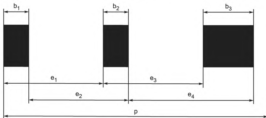
Рисунок 5 — Декодирование размеров
