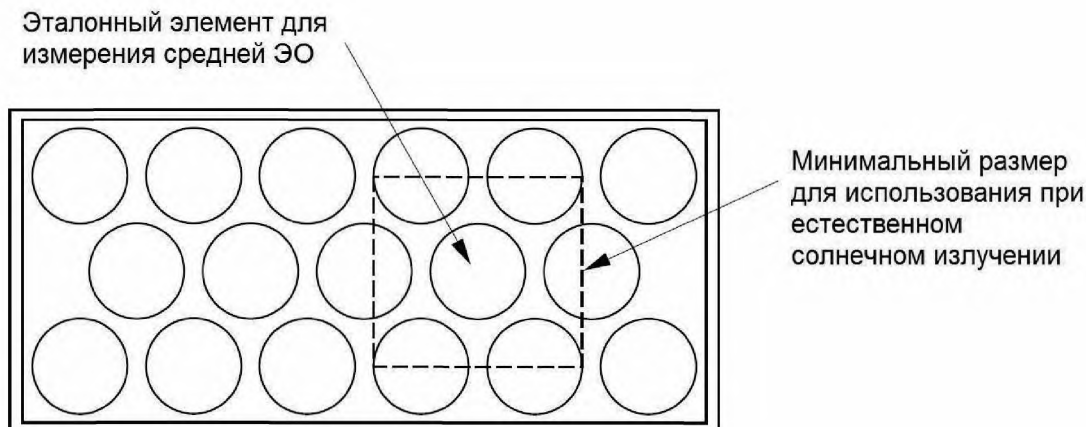
Рисунок 1 – Пример эталонного солнечного элемента в многоэлементном корпусе
