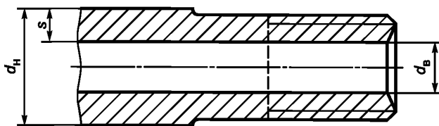
Рисунок 1 — Элемент трубы
