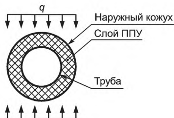
Рисунок 12.1 — К определению жесткости поперечного сечения на изгиб
