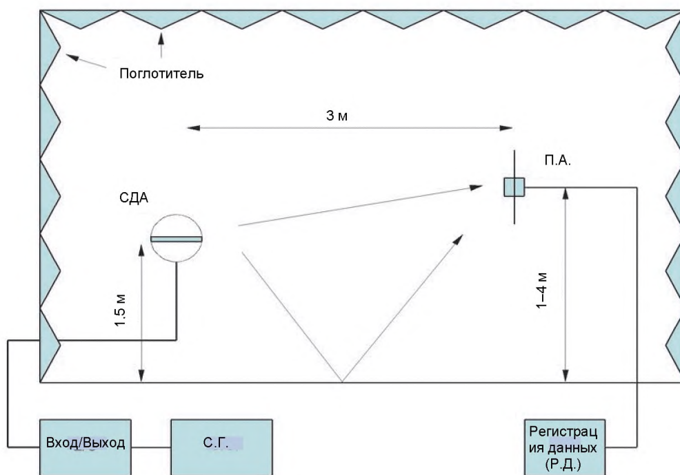
Рисунок А.3 в – Система измерения в месте испытаний объекта измерения
