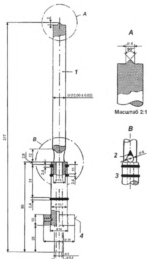
1 – внутренний электрод; 2 – отметка заполнения; 3 – уплотнительные кольца внешним диаметром 16,1 мм и внутренним диаметром 11,3 мм; 4 – рифленая поверхность
