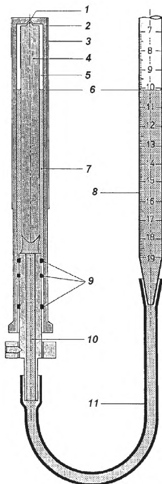
1 – центрирующий конус; 2 – стеклянная реакционная камера; 3 – наружный электрод (фольга А1); 4 – внутренний электрод; 5 – газовый карман; 6 – уровень масла; 7 – проба масла; 8 – бюретка; 9 – уплотнительные кольца; 10 – масляный канал; 11 – соединительная трубка
