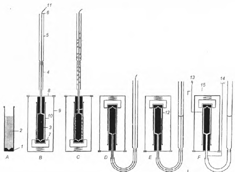
А – заполнение реакционной камеры пробой масла (уровень заполнения); В – введение внутреннего электрода (с соединительным шлангом, бюреткой и капиллярной трубкой); С – насыщение испытательным газом; D – перевертывание держателя вверх ногами (положение при испытании); Е – подача испытательного газа через капиллярную трубку; F – размещение испытательной установки в масляной бане, подача напряжения; 1 – стеклянная реакционная камера; 2 – испытуемое масло; 3 – внутренний электрод; 4 – соединительная трубка; 5 – бюретка; 6 – капиллярная трубка; 7 – подпружиненная упорная пластина; 8 – стопор; 9 – держатель; 10 – наружный электрод; 11 – подача газа; 12 – испытательный газ; 13 – высоковольтные провода; 14 – заземление; 15 – масляная баня
