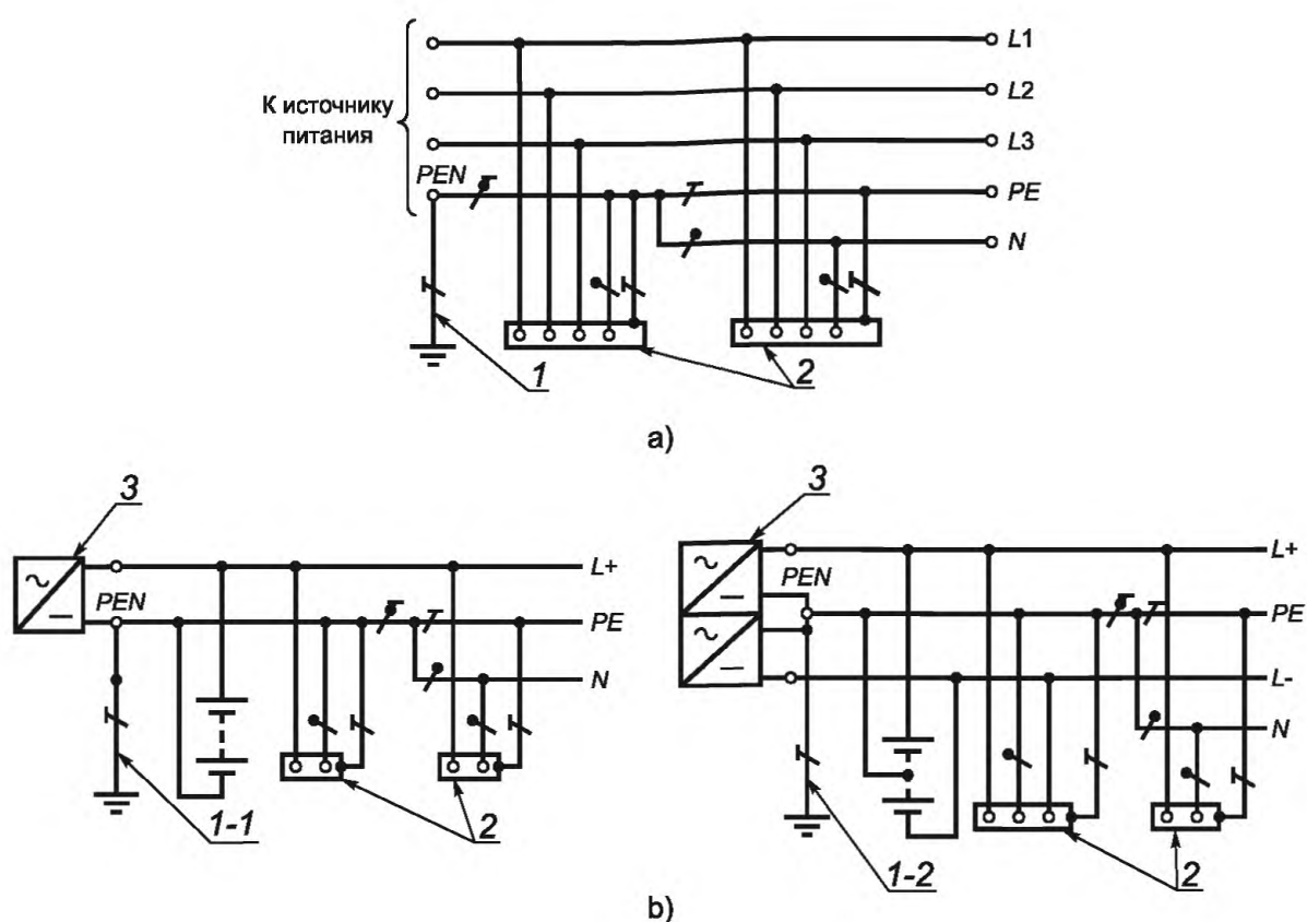
Рисунок 2 — Система TN-S переменного (а) и постоянного (б) тока. Нулевой защитный и нулевой рабочий проводники разделены
