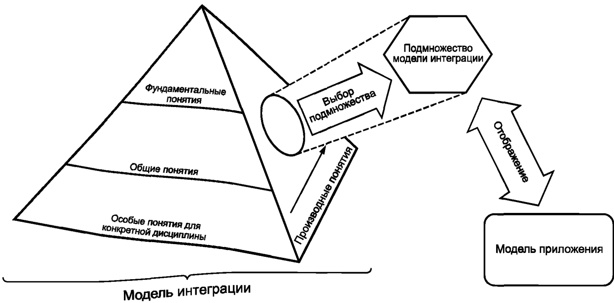
Рисунок 9 — Интеграция моделей приложений с моделью интеграции
