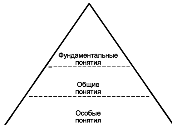
Рисунок 7 — Примитивные понятия
