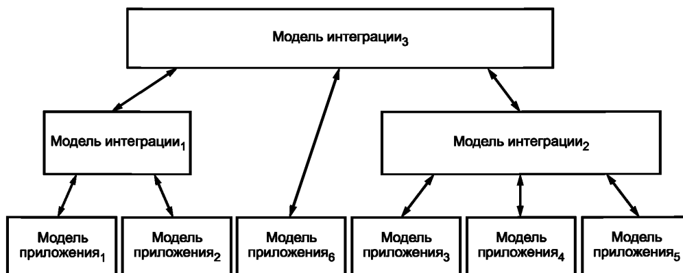
Рисунок 1 — Модель интеграции
